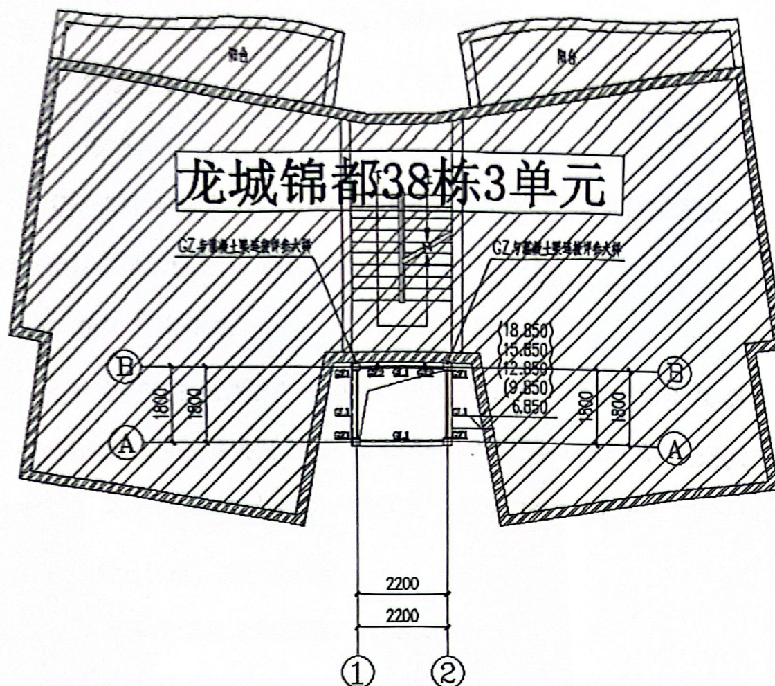
图 2-1 新增电梯标准层结构平面布置
