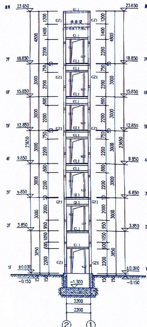
②-①轴立面图 1:100 电梯承重量应结合电梯工艺图定位
