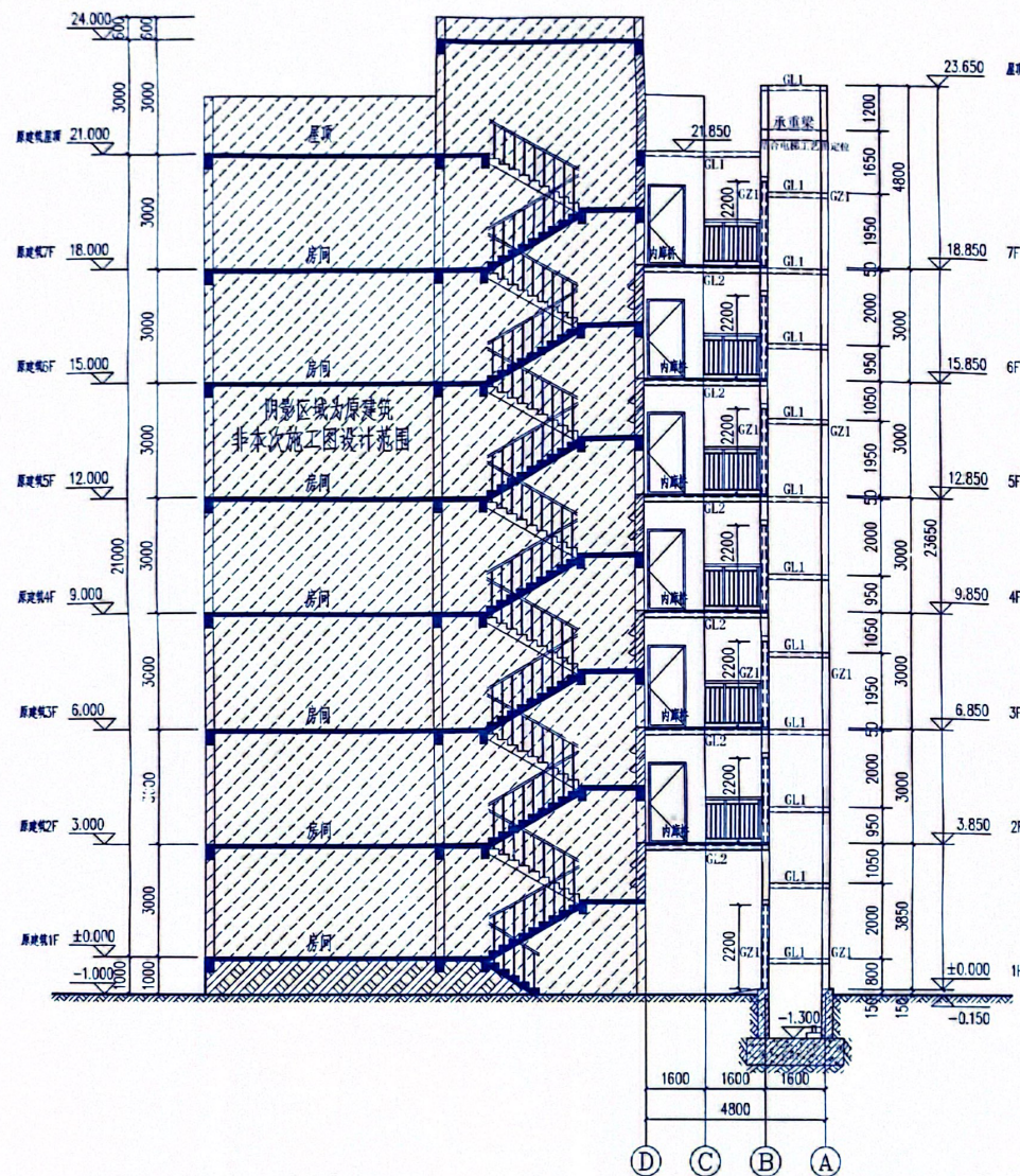
1-1剖面图 1:100
