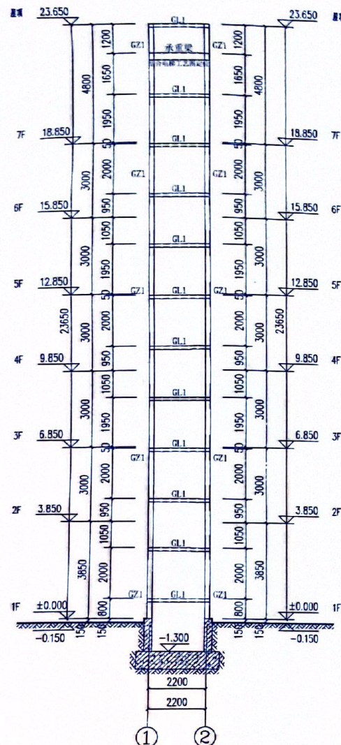
①-②轴立面图 1:100 电梯承重量应结合电梯工艺图定位
