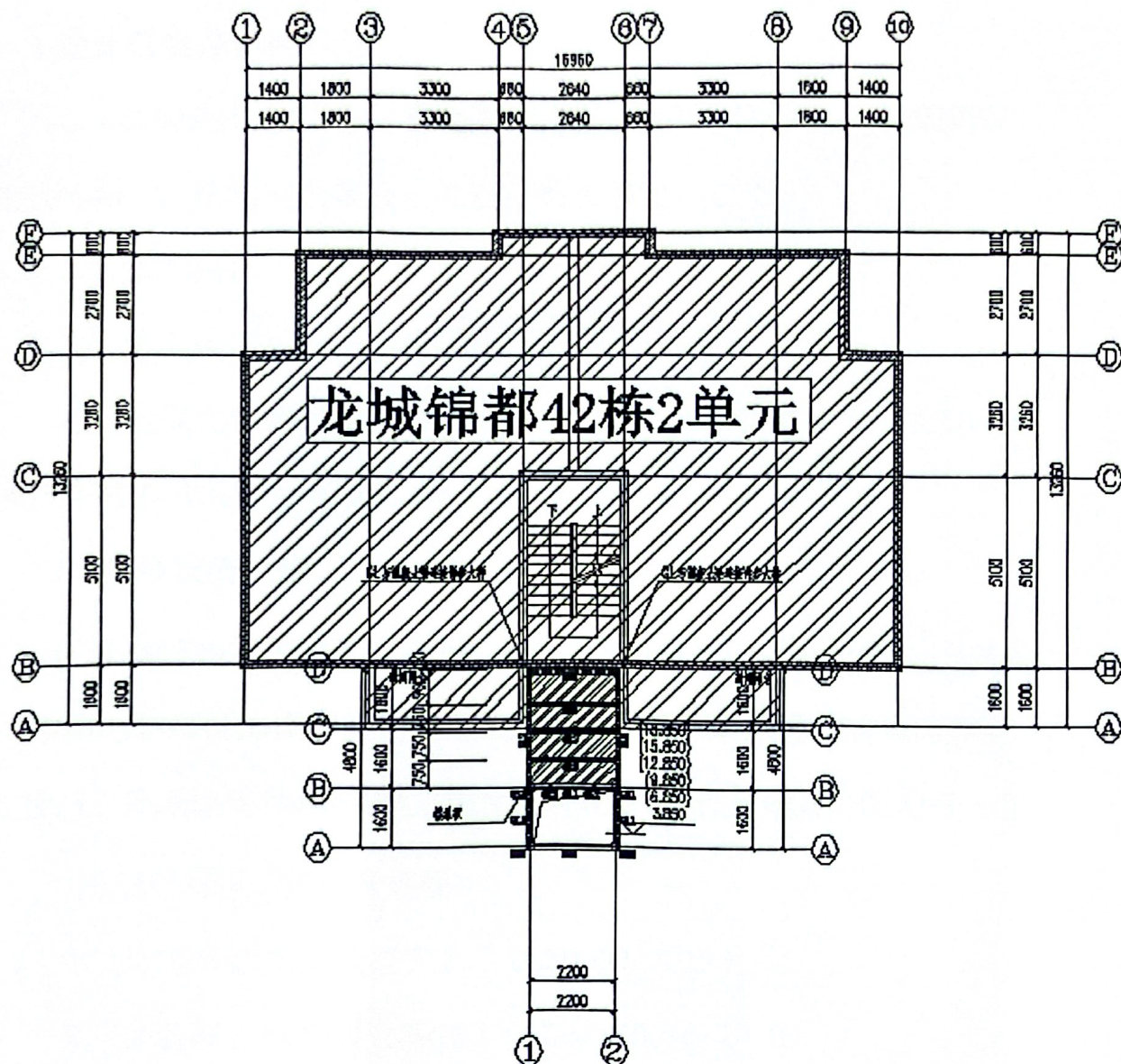
图 2-1 新增电梯标准层结构平面布置
