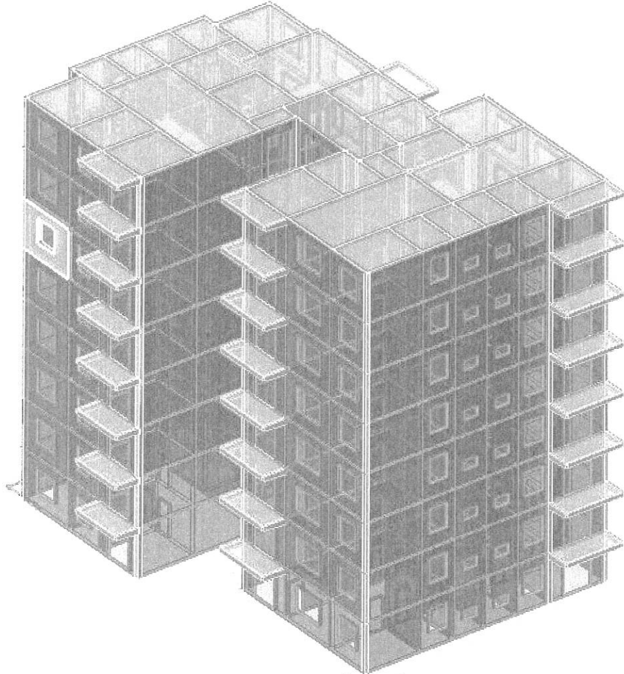
图 6-1 验算模型
