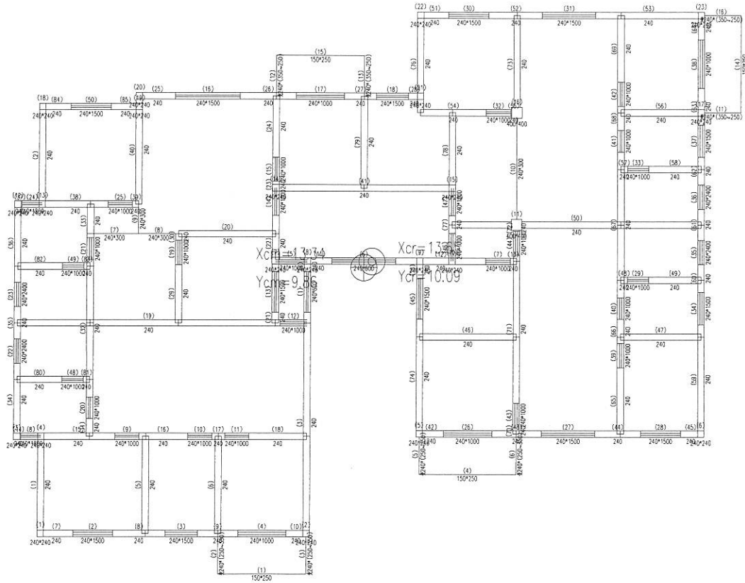
第 7 层设计模型构件编号简图 (红色代表本层核心筒、黄色代表梁/墙/柱合模心、绿色代表楼梯合模心坐标)
