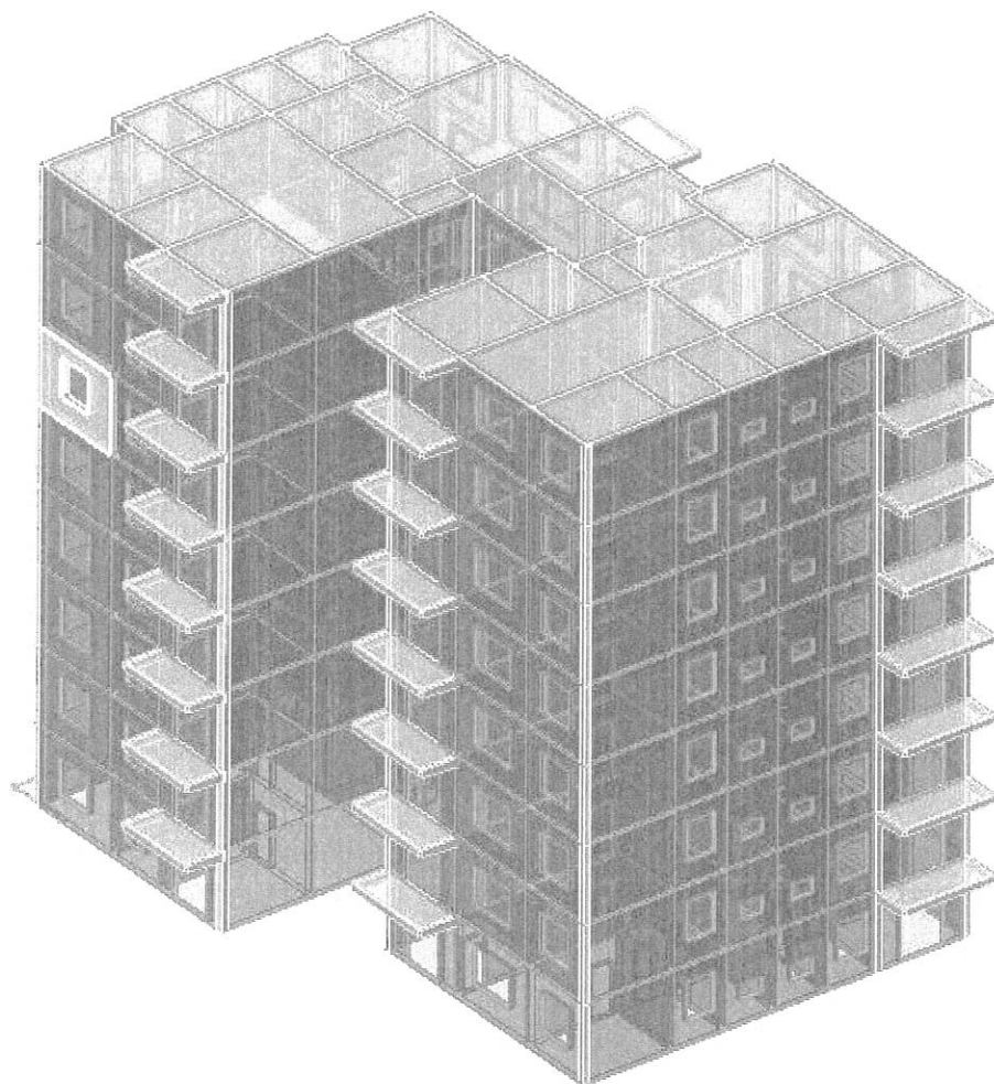
图 4-1 结构三维模型图
