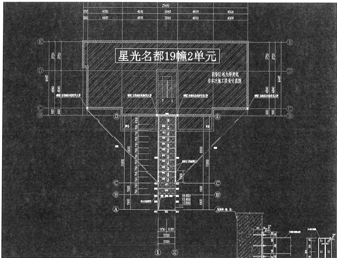
图 2-1 新增电梯标准层结构平面布置
