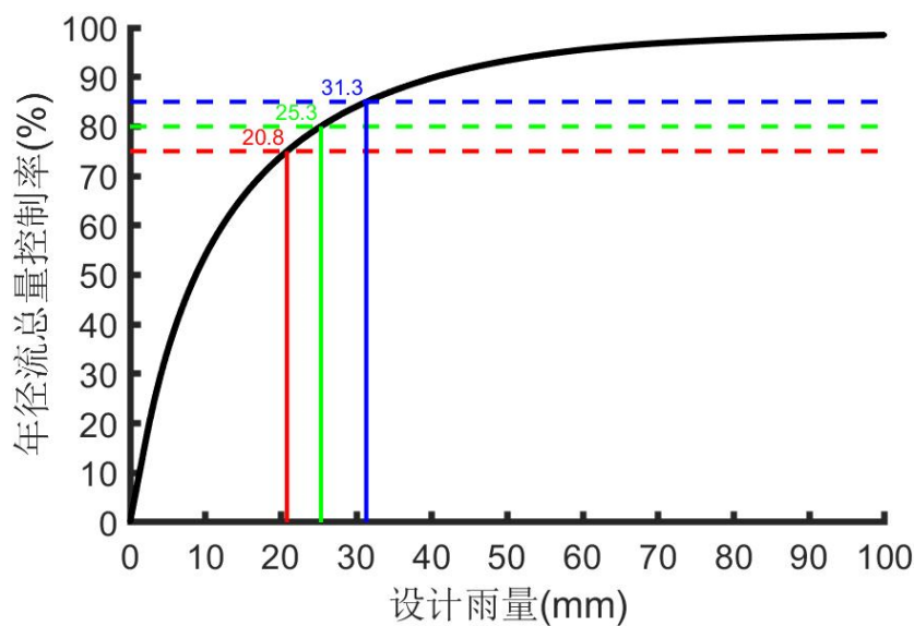
图 5.4-7 园区不同年径流控制率对应的设计降雨量
