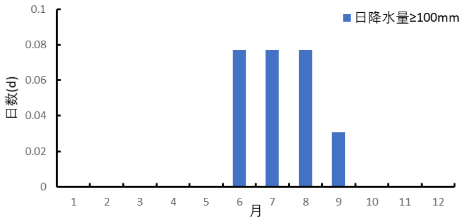
图 5.4-3b 日降水量≥100.0mm 平均日数的年变化(1955~2019 年)
