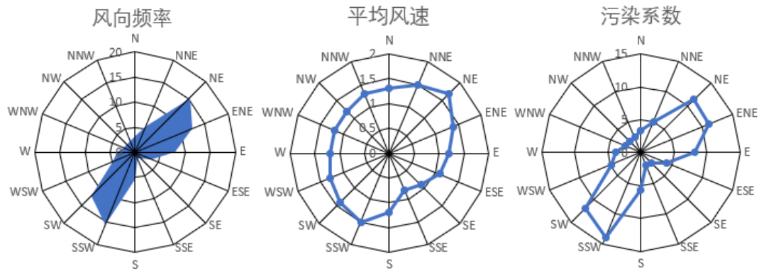
图 5.7-3 秋季风向频率、平均风速及污染系数分布(2010~2019 年)
