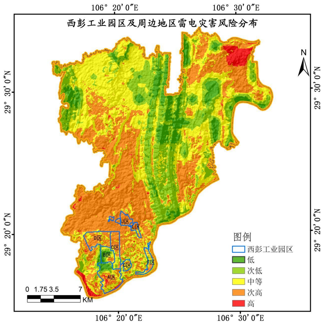
图 6.4-17 西彭工业园区及周边地区雷电灾害风险分布
