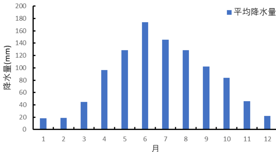
图 3.5-2 参证站年降水量年变化(1990~2019 年)
