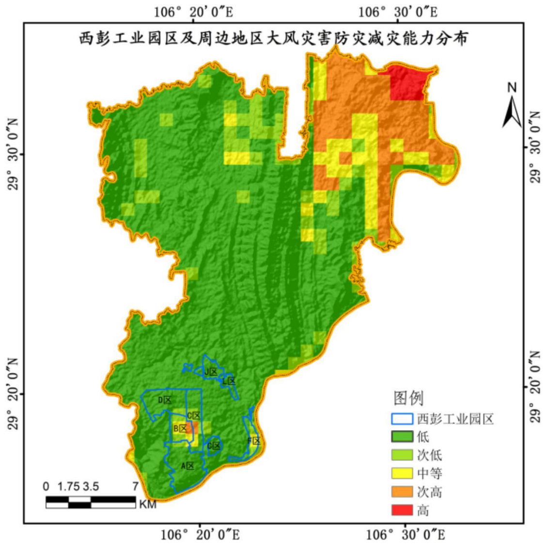
图 6.2-4 西彭工业园区及周边地区大风灾害防灾减灾能力分布
