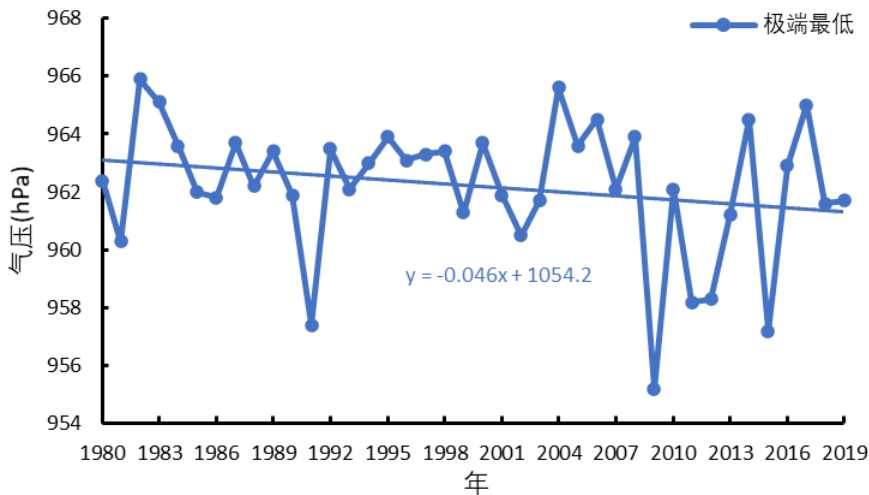
图 3.2-3 参证站极端最低气压年际变化(1980~2019 年)
