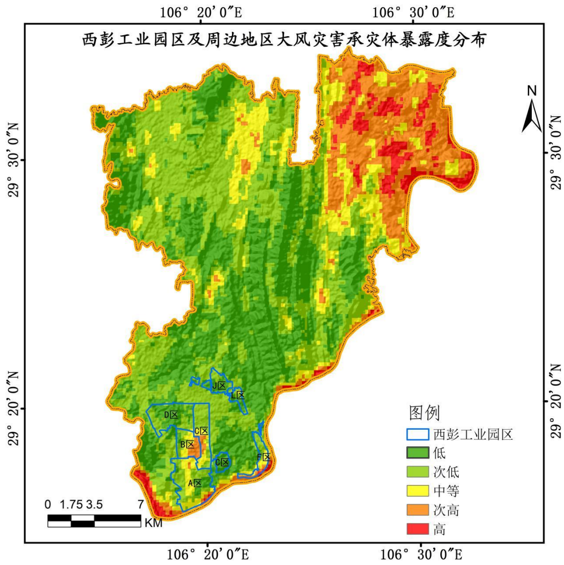
图 6.2-2 西彭工业园区及周边地区承灾体暴露度分布
