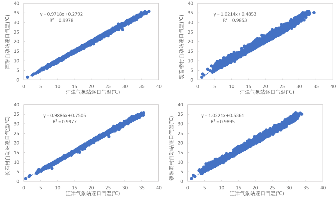
图 2.4-2 江津气象站与园区周边自动站逐日平均气温相关图(2013~2019 年)
