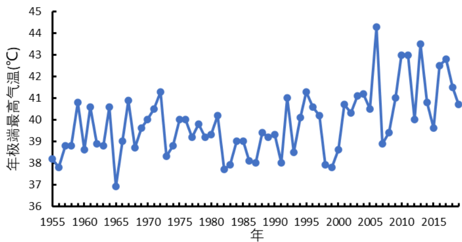
图 5.2-2 参证站年极端最高气温年际变化(1955~2019 年)
