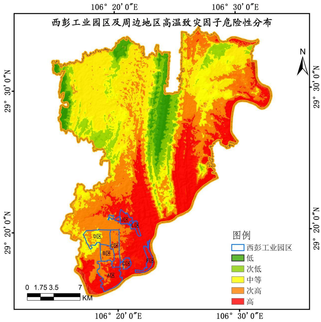
图 6.1-1 西彭工业园区及周边地区高温致灾因子危险性空间分布
