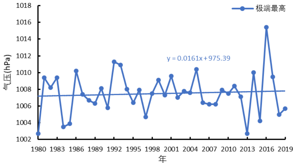
图 3.2-2 参证站极端最高气压年际变化(1980~2019 年)
