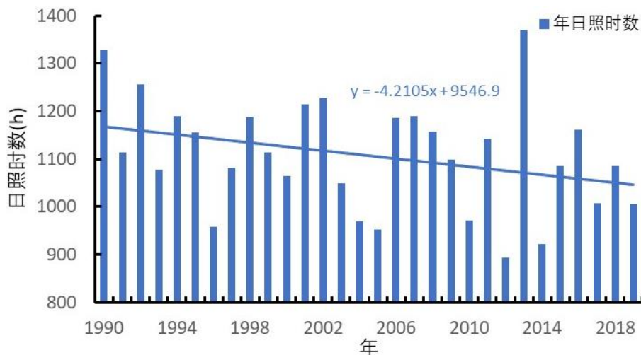
图 3.7-1 参证站年日照时数年际变化(1990~2019 年)
