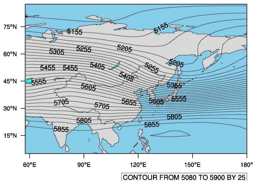
图 3.1-1 春季 500hPa 平均环流场(1990-2019 年)
