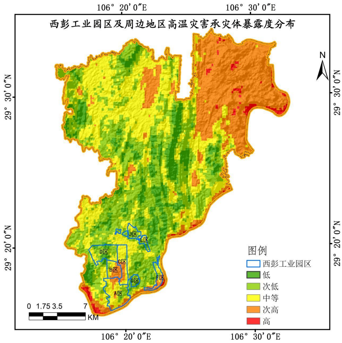
图 6.1-2 西彭工业园区及周边地区高温承灾体暴露度空间分布
