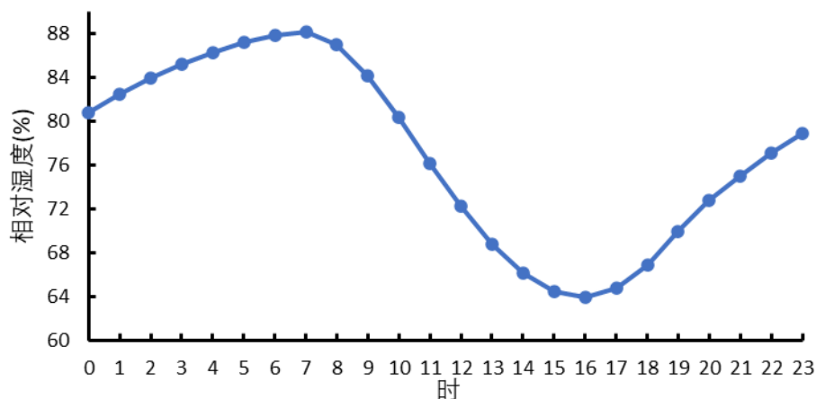
图 3.4-4 参证站平均相对湿度的日变化(2010~2019 年)
