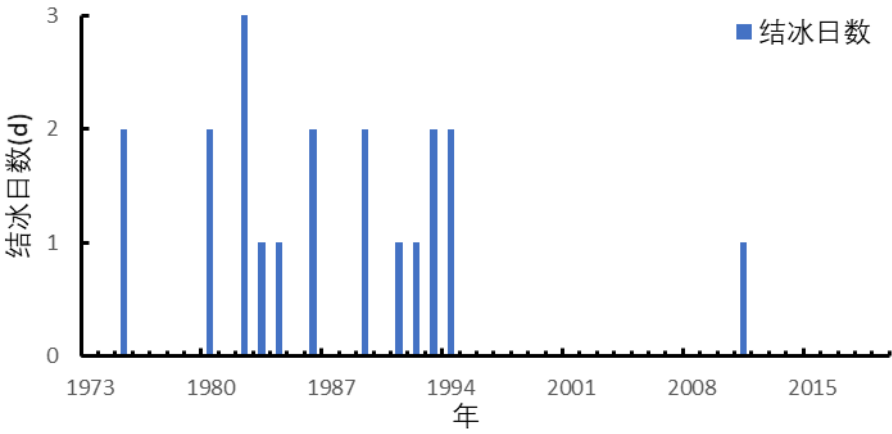
图 4.6-1 参证站结冰日数年际变化(1973~2019 年)
