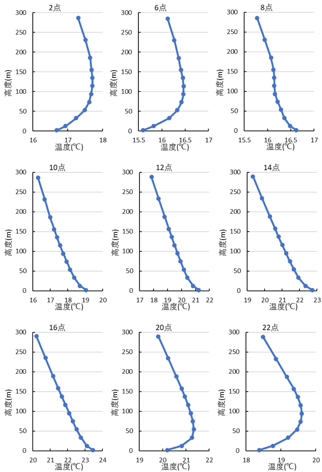
图 5.3-9 西彭工业园区各时刻平均气温随高度变化曲线
