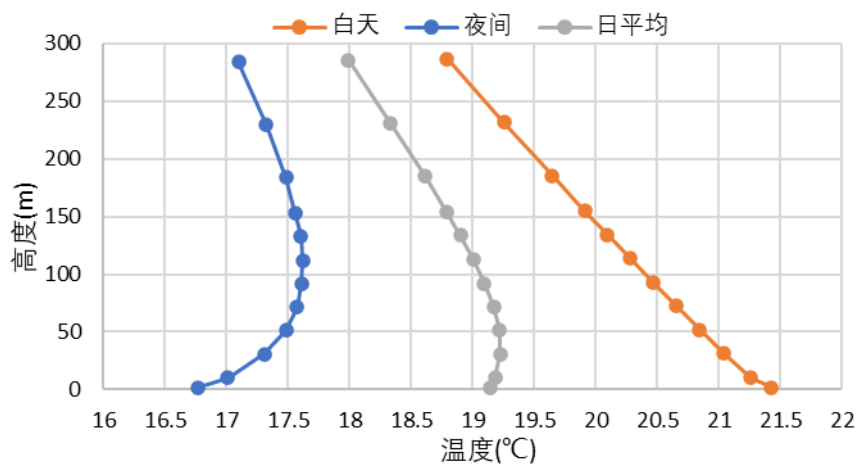
图 5.3-10 西彭工业园区低空白天、夜间和日平均气温随高度变化曲线
