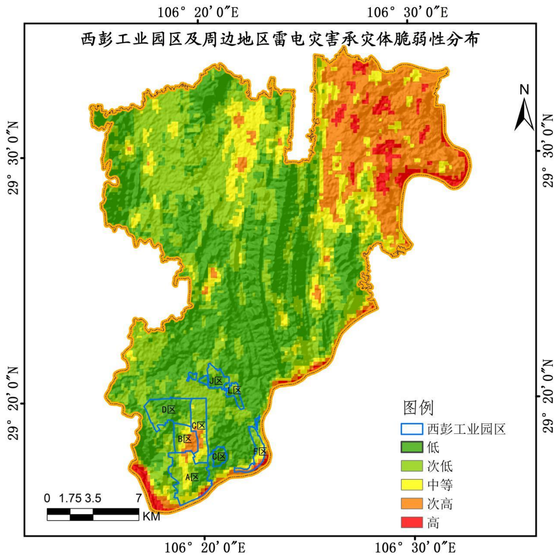
图 6.4-15 西彭工业园区及周边地区雷电灾害承灾体脆弱性
