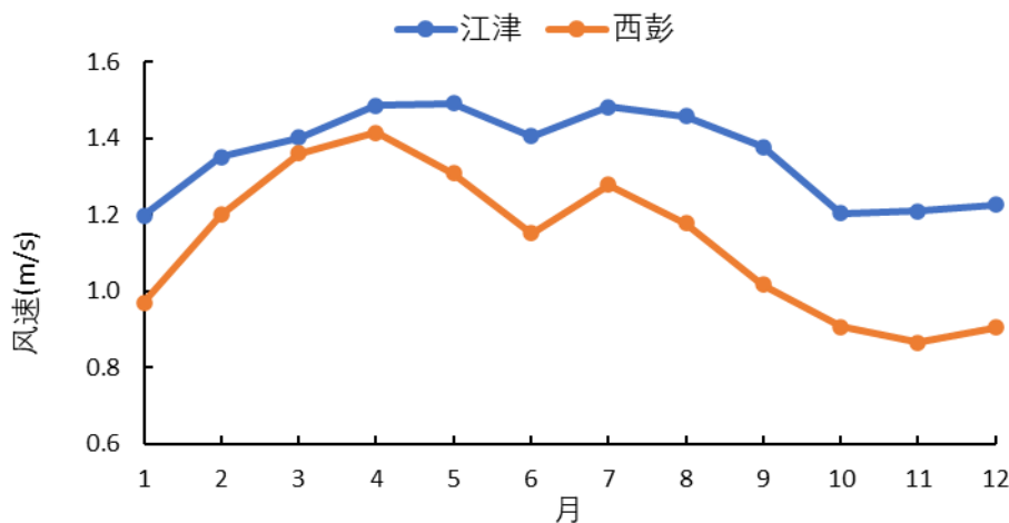
图 2.4-4 江津气象站与西彭自动站平均风速年变化(2013~2019 年)
