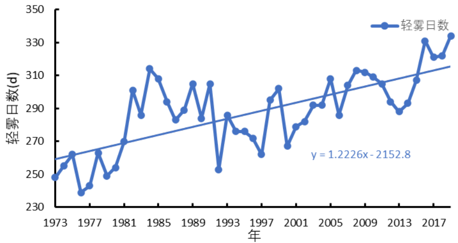
图 4.8-1 参证站累年轻雾日数年际变化(1973~2019 年)
