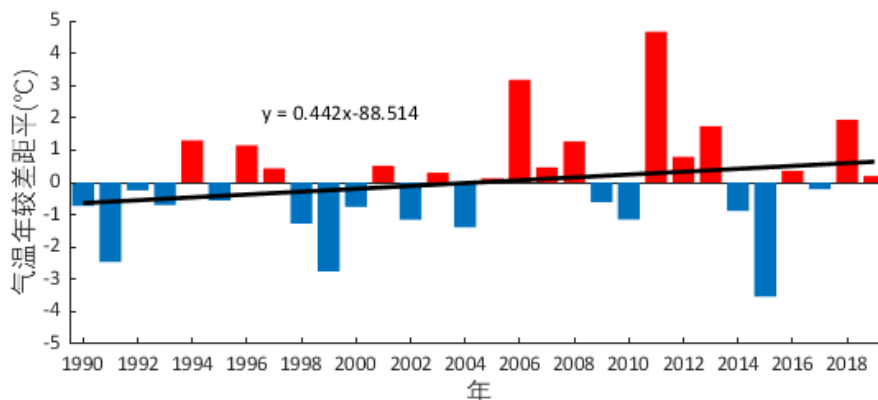
图 3.3-2 参证站平均气温年较差距平年际变化(1990~2019 年)
