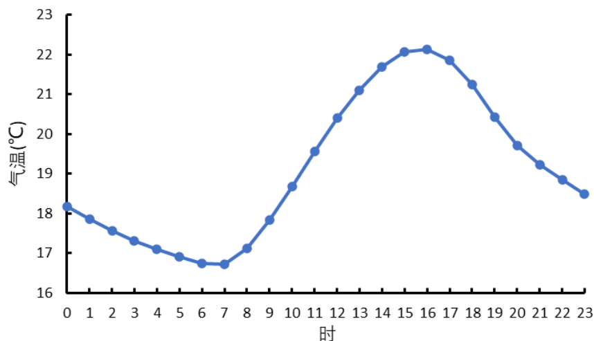
图 3.3-6 参证站平均气温的日变化(2010~2019 年)
