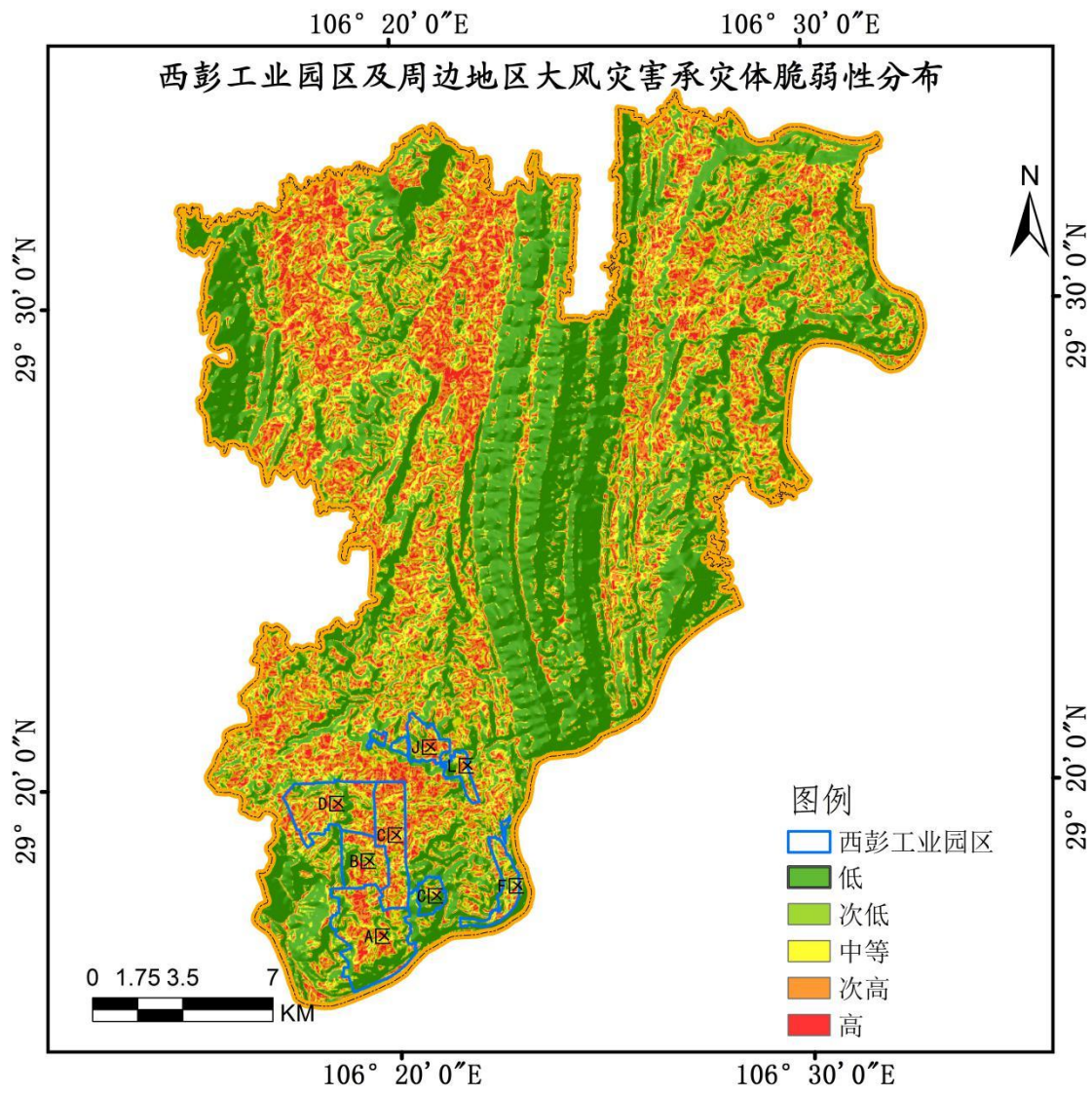
图 6.2-3 西彭工业园区及周边地区大风承灾体脆弱性分布
