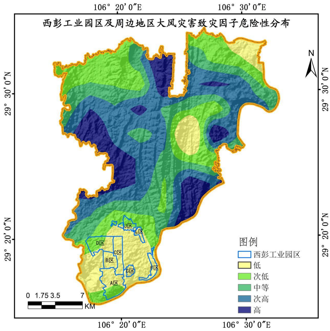
图 6.2-1 西彭工业园区及周边地区大风灾害致灾因子危险性分布
