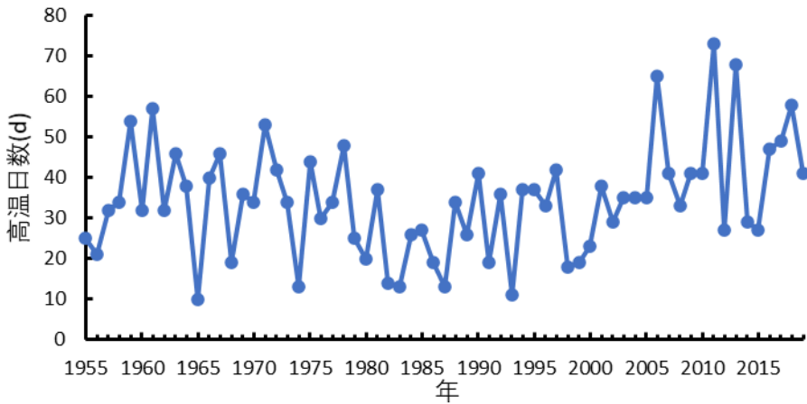
图 5.2-4 参证站高温日数年际变化图(1955~2019 年)
