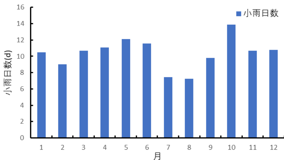
图 3.5-5 参证站小雨日数年变化(1990~2019 年)
