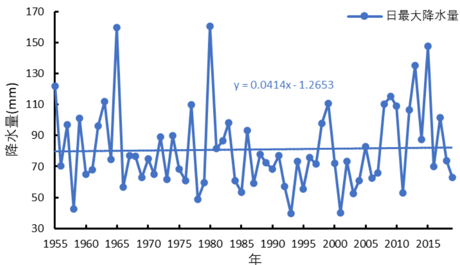
图 4.3-1 参证站日最大降水量年际变化(1955~2019 年)
