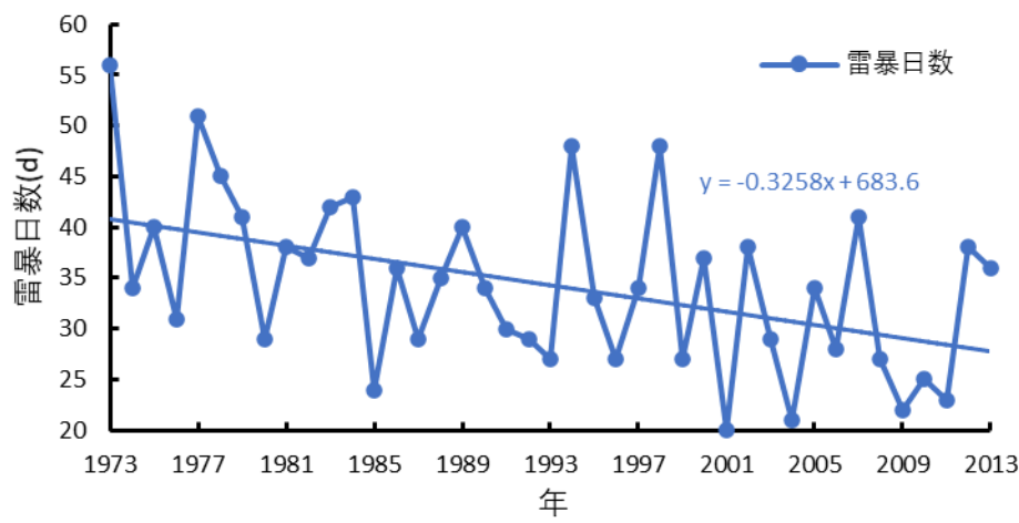
图 4.9-1 参证站雷暴日数年际变化(1973~2013 年)
