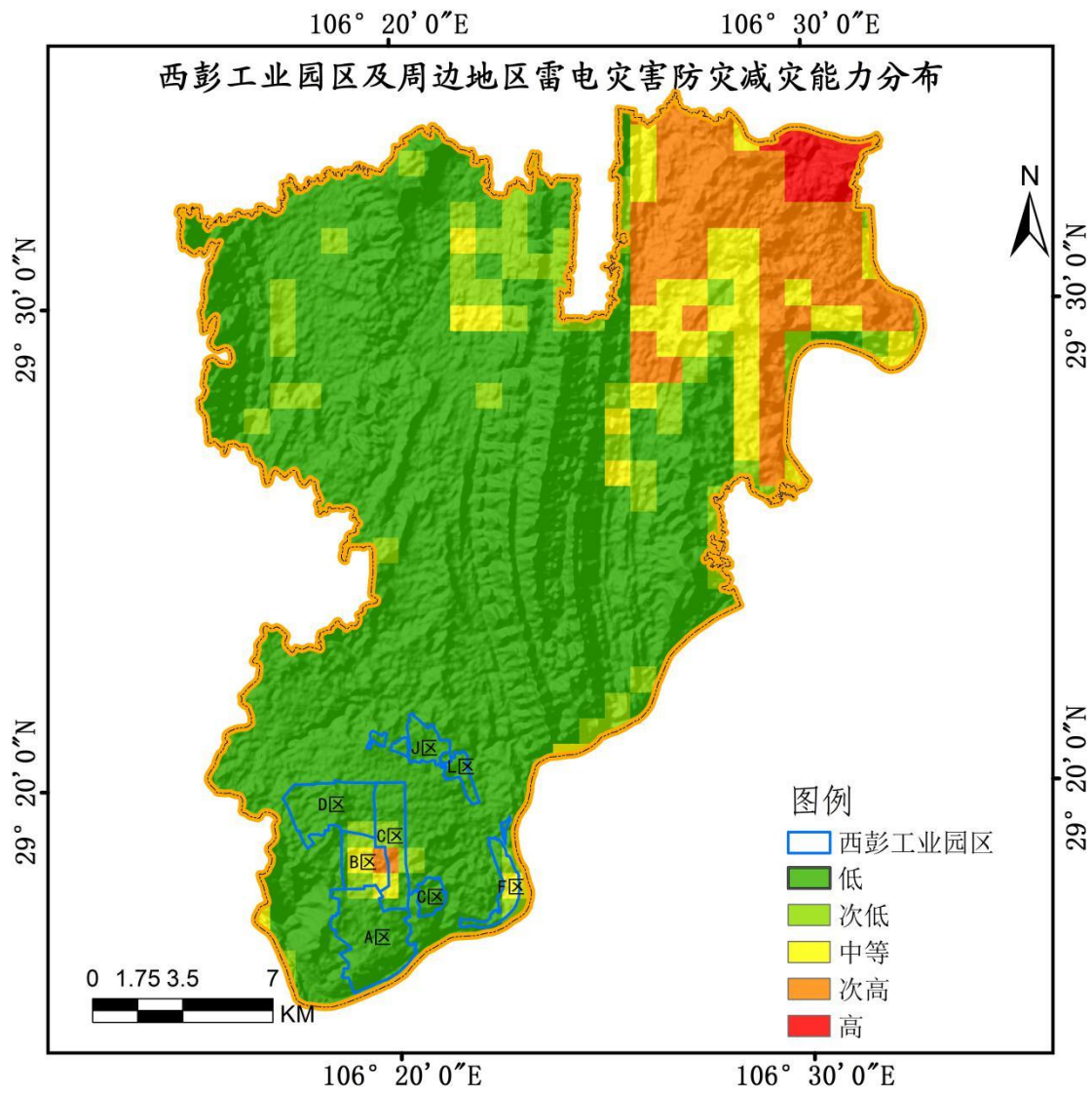
图 6.4-16 西彭工业园区及周边地区雷电防灾减灾能力
