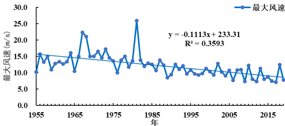
图 3.8-2 参证站年最大风速年际变化(1955~2019 年)
