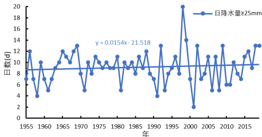
图 5.4-1a 日降水量 \geq 25.0\text{mm} 日数的年际变化(1955~2019 年)
