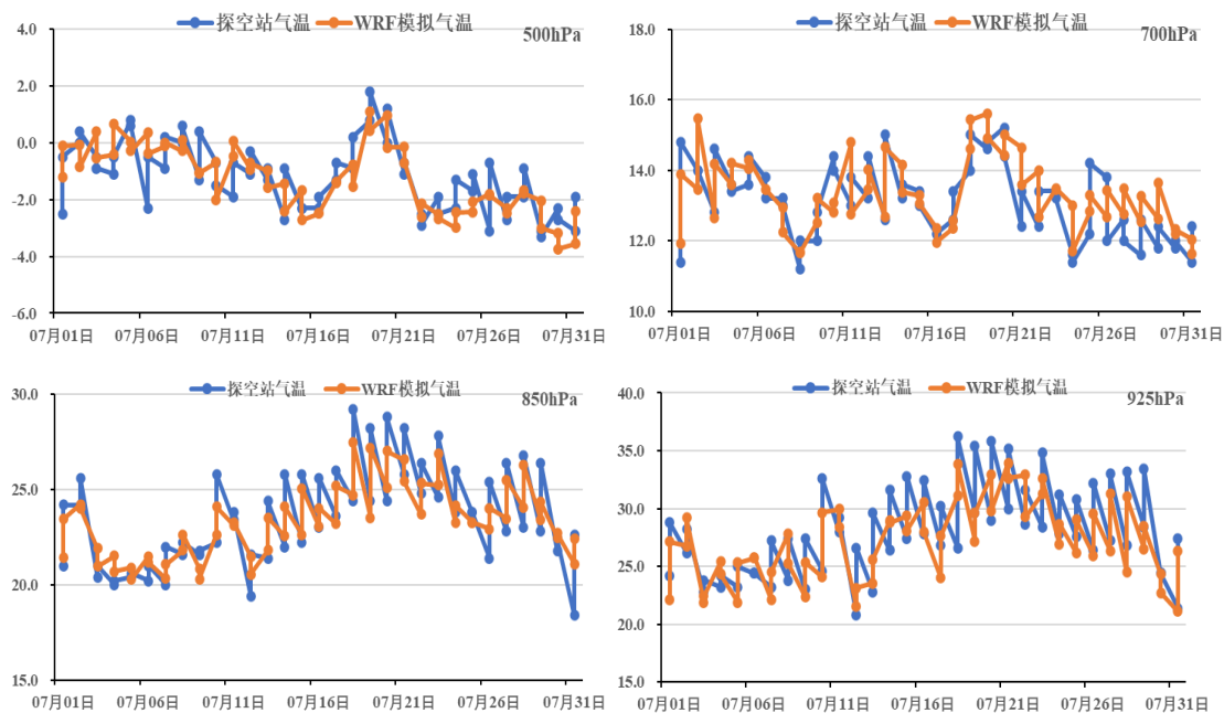
图 5.3-6 7 月模拟气温与探空站气温对比
