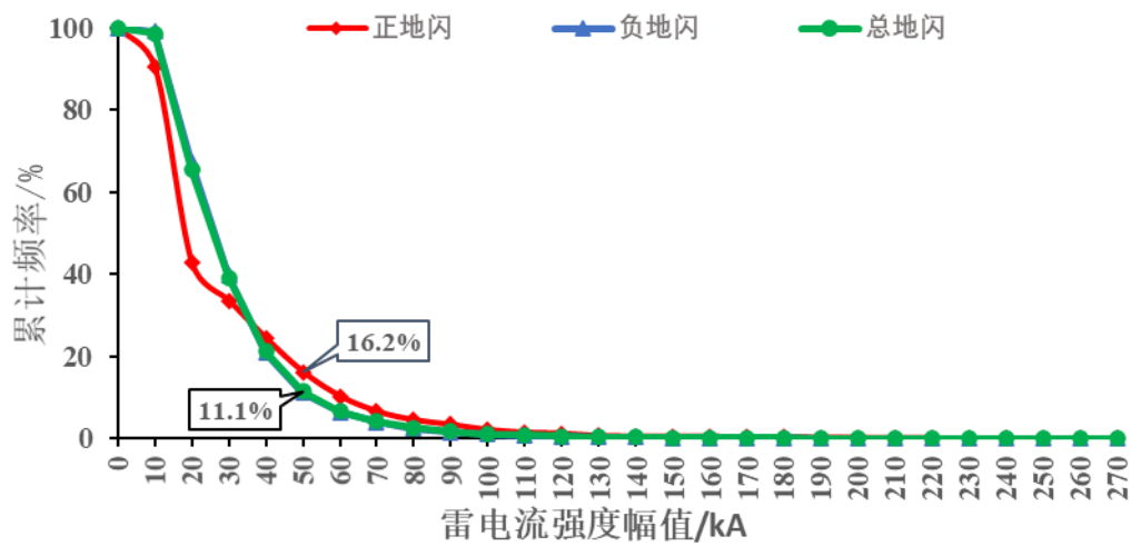
图 6.4-11 园区及周边雷电流强度幅值累积频率分布（2010~2019 年）
