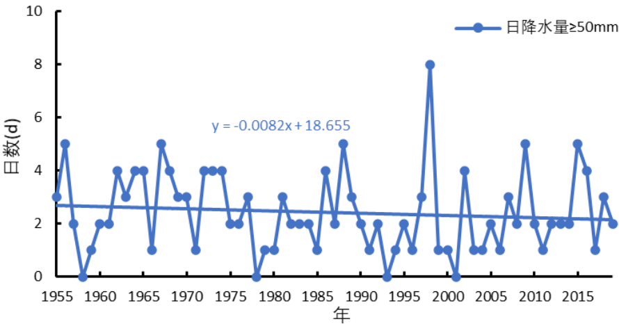
图 5.4-2a 日降水量 \geq 50.0\text{mm} 日数的年际变化(1955~2019 年)
