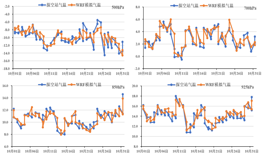
图 5.3-7 10 月模拟气温与探空站气温对比
