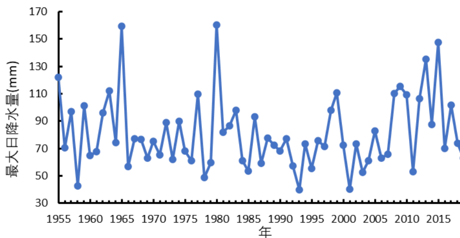
图 5.2-1 参证站最大日降水量年际变化(1955~2019 年)
