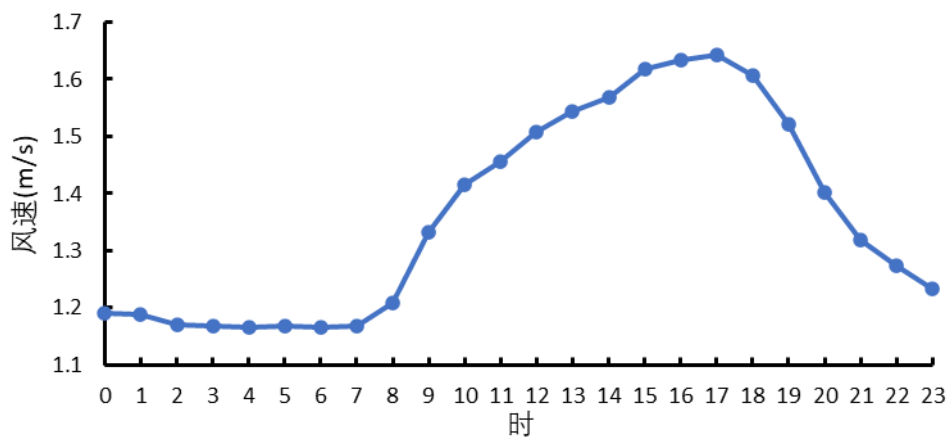
图 3.8-5 参证站平均风速日变化(2010~2019 年)
