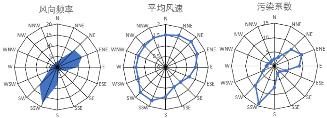
图 5.7-2 夏季风向频率、平均风速及污染系数分布(2010~2019 年)
