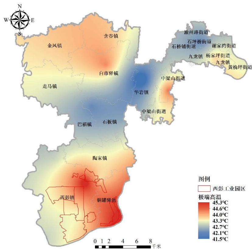
图 4.2-2 九龙坡极端最高气温空间分布图(2013~2019 年)
