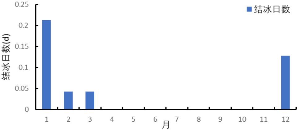
图 4.6-2 参证站结冰日数年变化(1973~2019 年)
