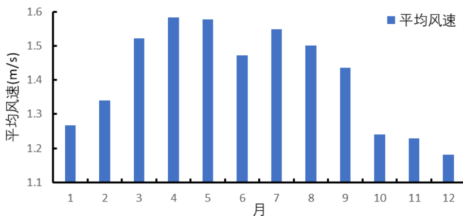
图 3.8-4 参证站平均风速年变化(1990~2019 年)
