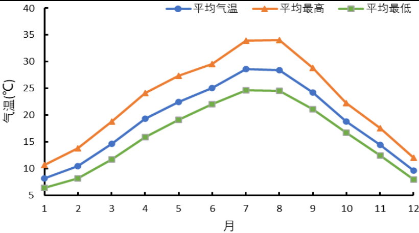
图 3.3-5 参证站平均气温、平均最高气温、平均最低气温年变化(1990~2019 年)
