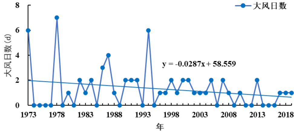
图 4.4-1 参证站大风日数年际变化(1973~2019 年)
