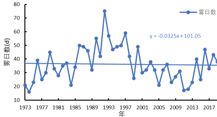
图 4.8-3 参证站雾日数年际变化(1973~2019 年)
