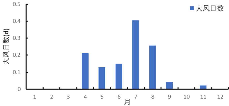
图 4.4-2 参证站大风日数年变化(1973~2019 年)
