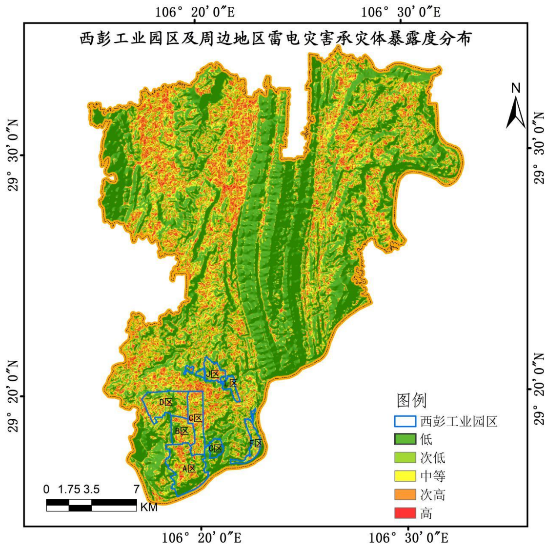
图 6.4-14 西彭工业园区及周边地区雷电承灾体暴露度分布
