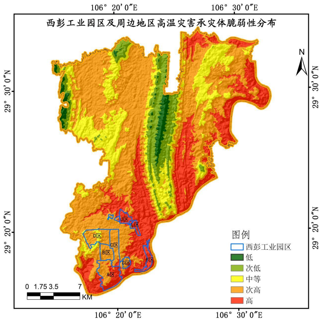
图 6.1-3 西彭工业园区及周边地区高温灾害承灾体脆弱性空间分布
