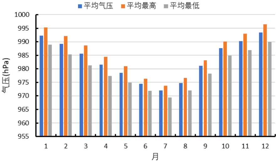
图 3.2-4 参证站平均气压、平均最高气压、平均最低气压年变化（1990~2019 年）
