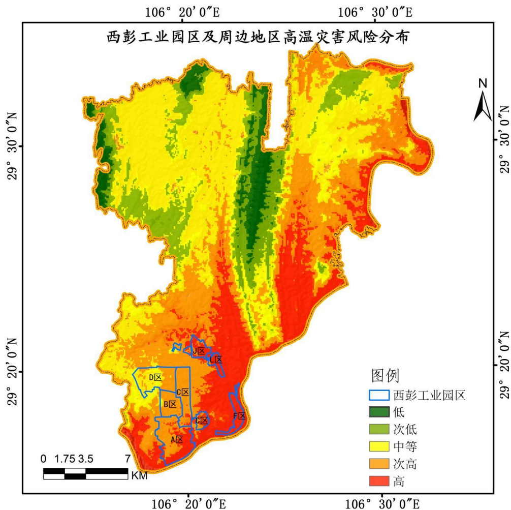
图 6.1-5 西彭工业园区及周边地区高温气象灾害风险分布
