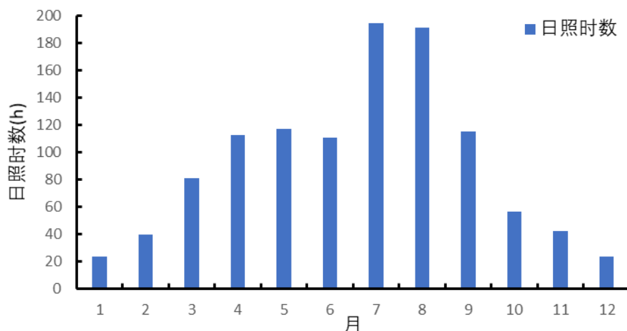
图 3.7-2 参证站平均日照时数年变化(1990~2019 年)
