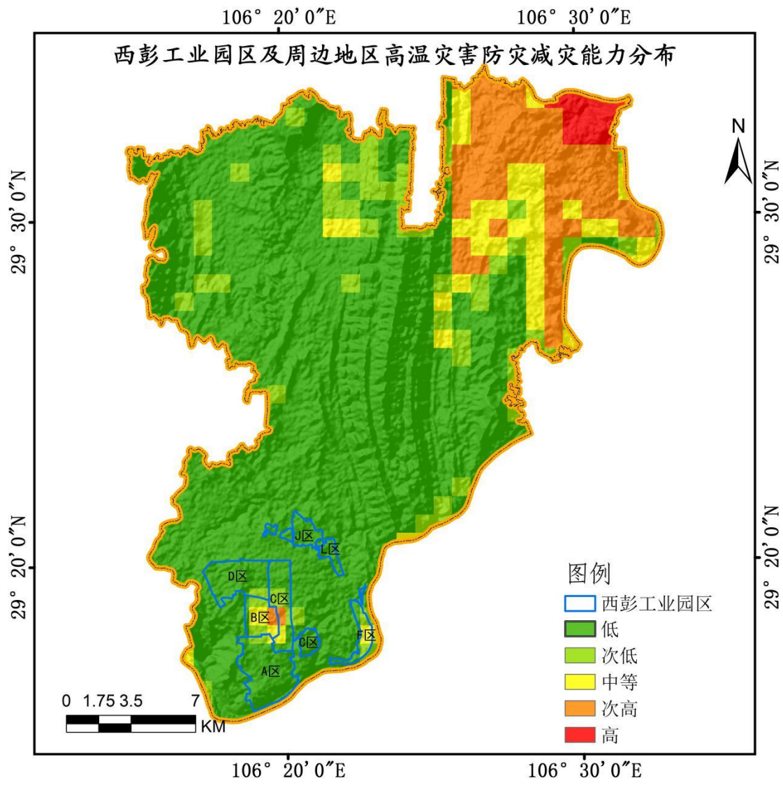
图 6.1-4 西彭工业园区及周边地区高温灾害防灾减灾能力分布
