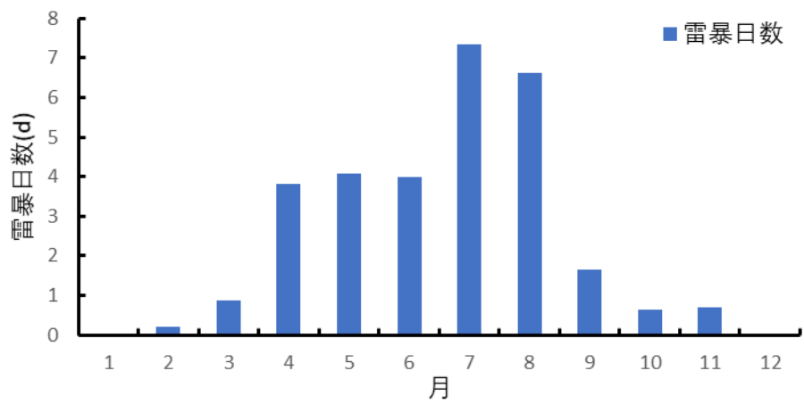
图 4.9-2 参证站累年雷暴日数年变化(1973~2013 年)
