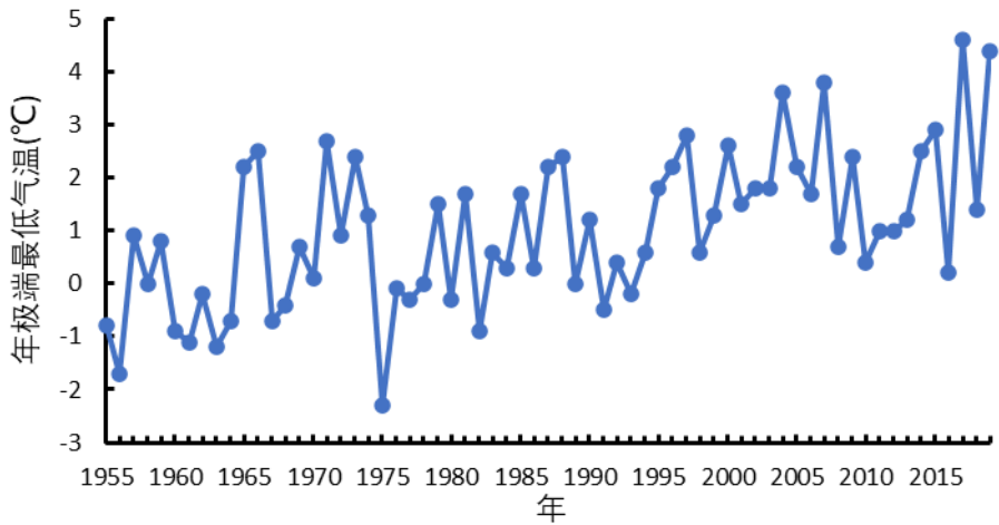
图 5.2-3 参证站年极端最低气温变化图(1955~2019 年)
