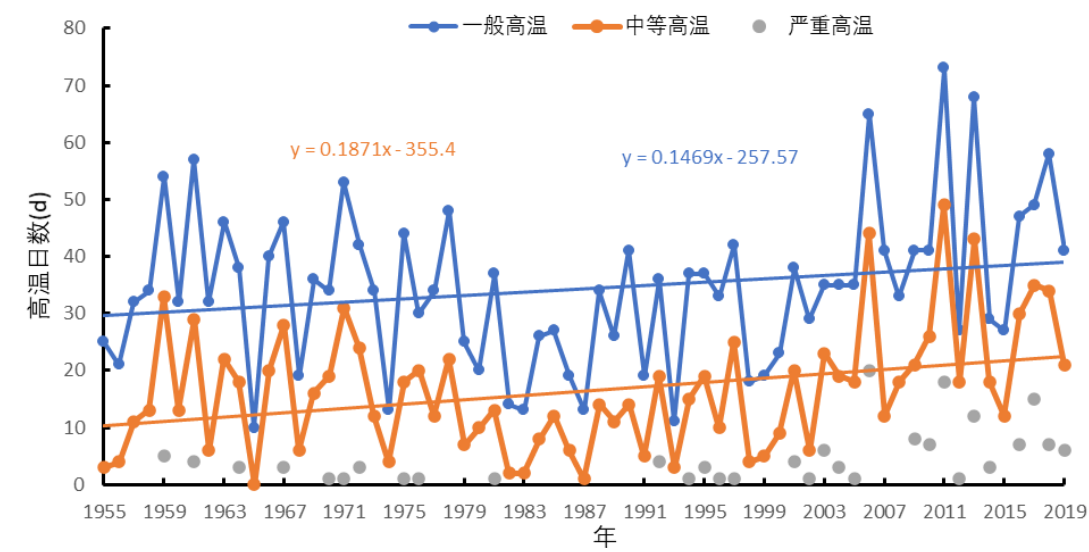
图 4.2-1 参证站累年高温日数年际变化(1955~2019 年)
