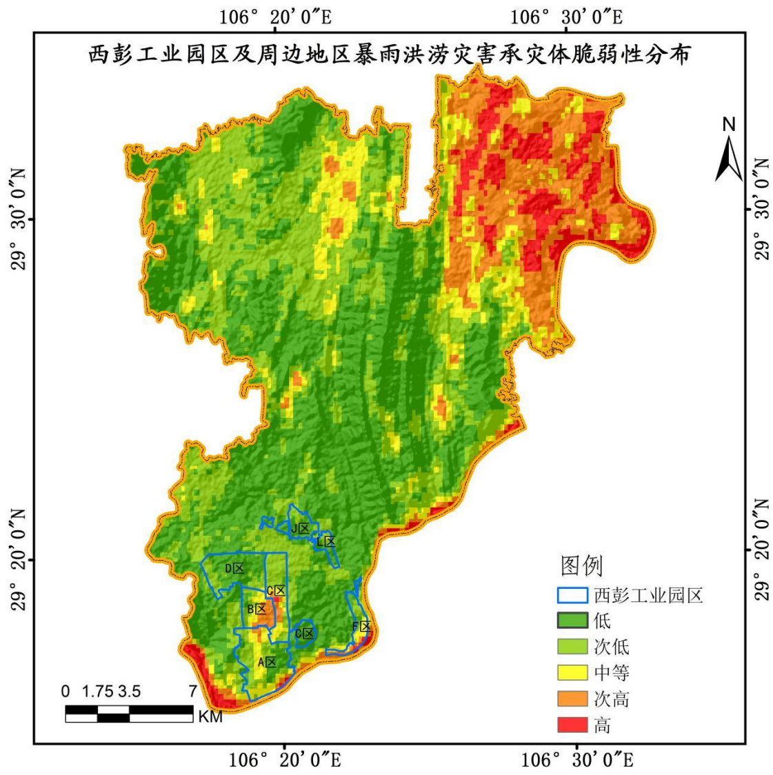
图 6.3-3 西彭工业园区及周边地区暴雨灾害承灾体脆弱性分布
