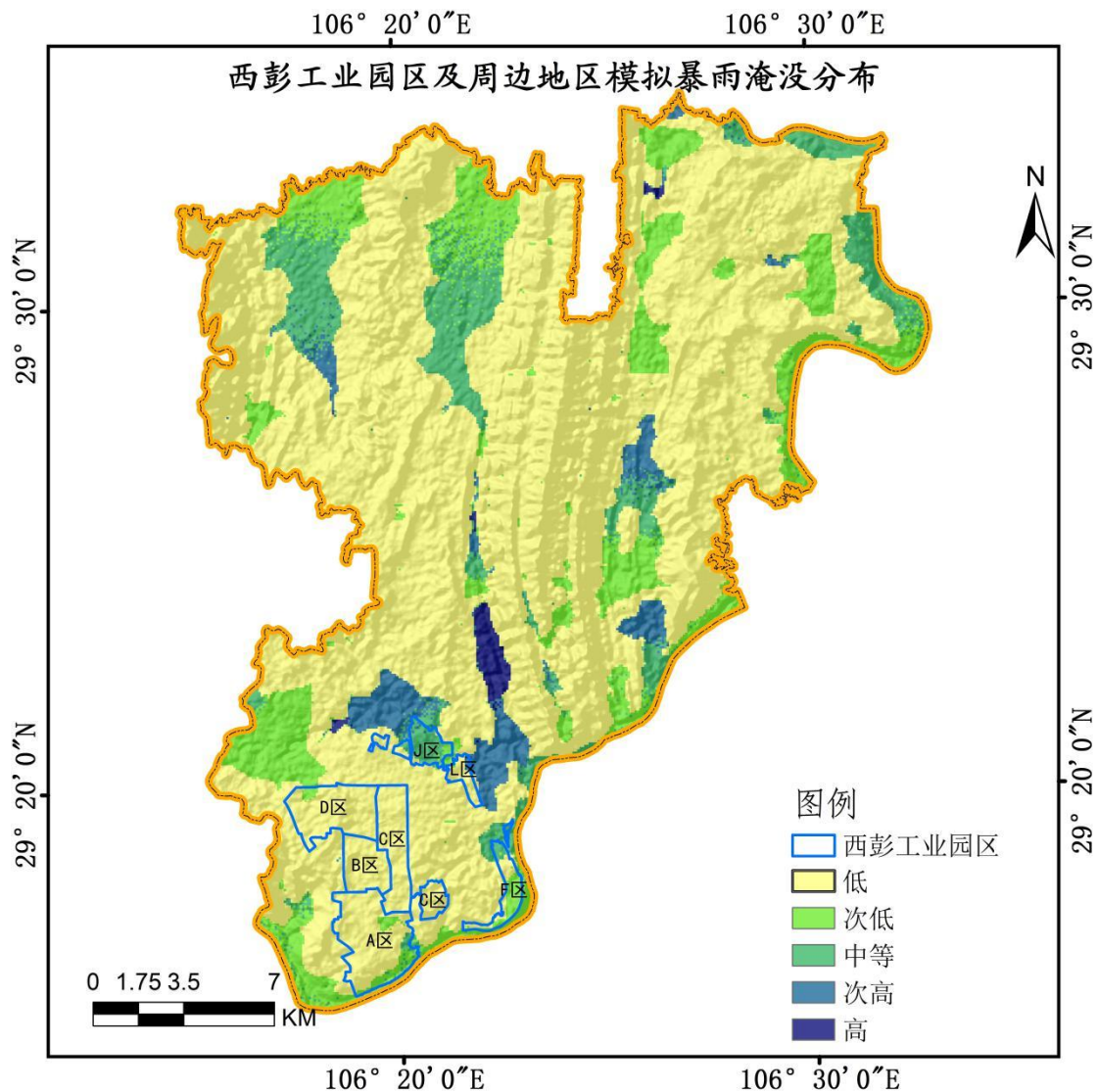
图 6.3-1 西彭工业园区及周边地区淹没水深模拟
