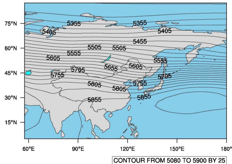
图 3.1-3 秋季 500hPa 平均环流场(1990-2019 年)
