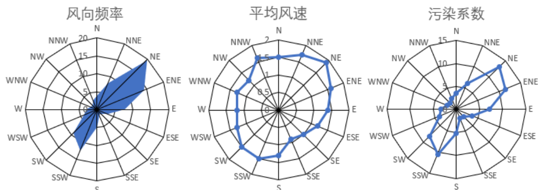
图 5.7-1 春季风向频率、平均风速及污染系数分布(2010~2019 年)
