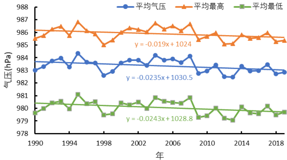
图 3.2-1 参证站年平均气压、平均最高气压、平均最低气压年际变化(1990~2019 年)
