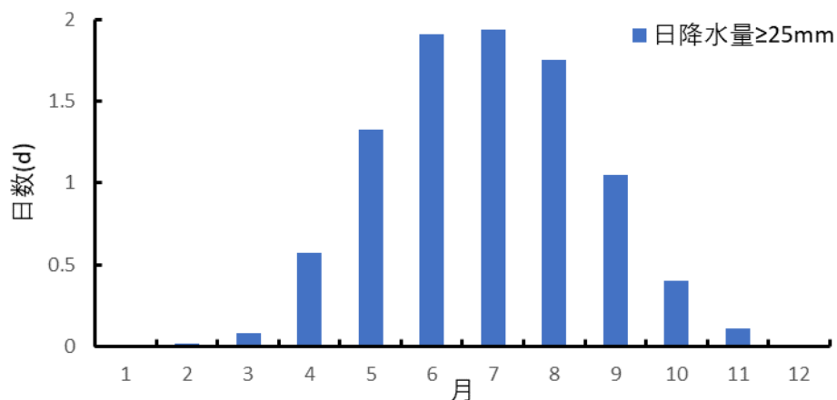
图 5.4-1b 日降水量 \geq 25.0\text{mm} 平均日数的年变化(1955~2019 年)
