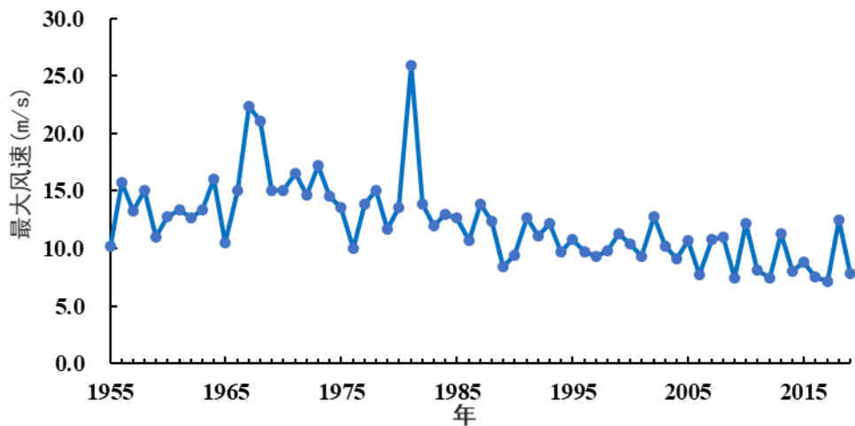
图 5.1-1 参证站订正后年最大风速年际变化
