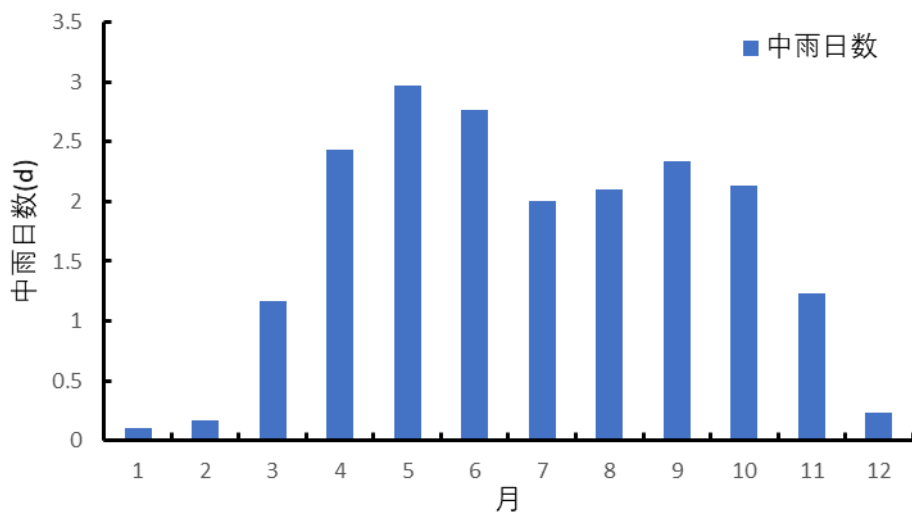
图 3.5-6 参证站中雨日数年变化(1990~2019 年)
