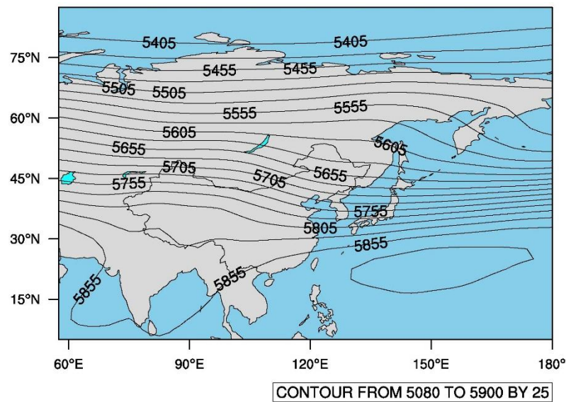
图 3.1-2 夏季 500hPa 平均环流场(1990-2019 年)
