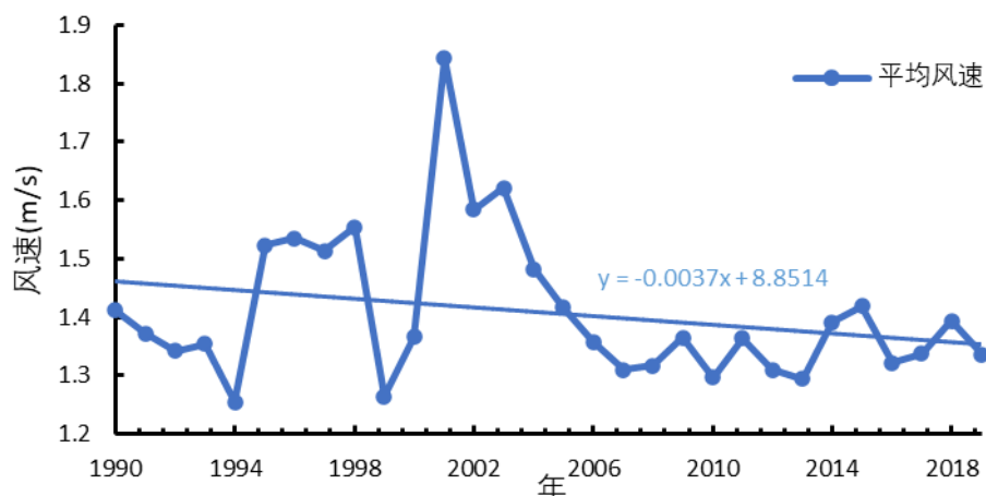
图 3.8-1 参证站年平均风速年际变化(1990~2019 年)
