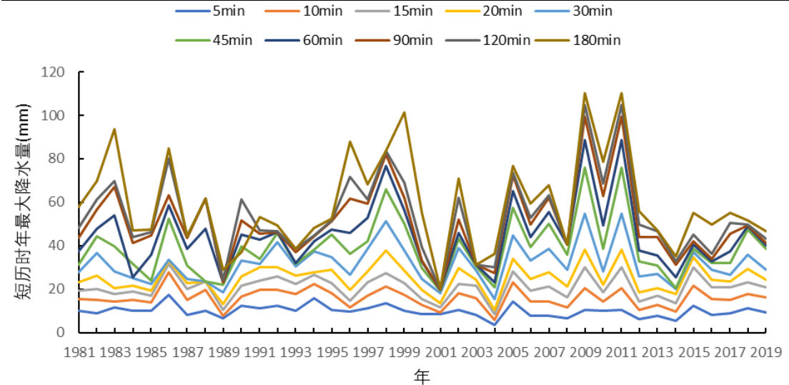
图 5.4-4 短历时年最大降水量年际的变化趋势图(1981~2019 年)
