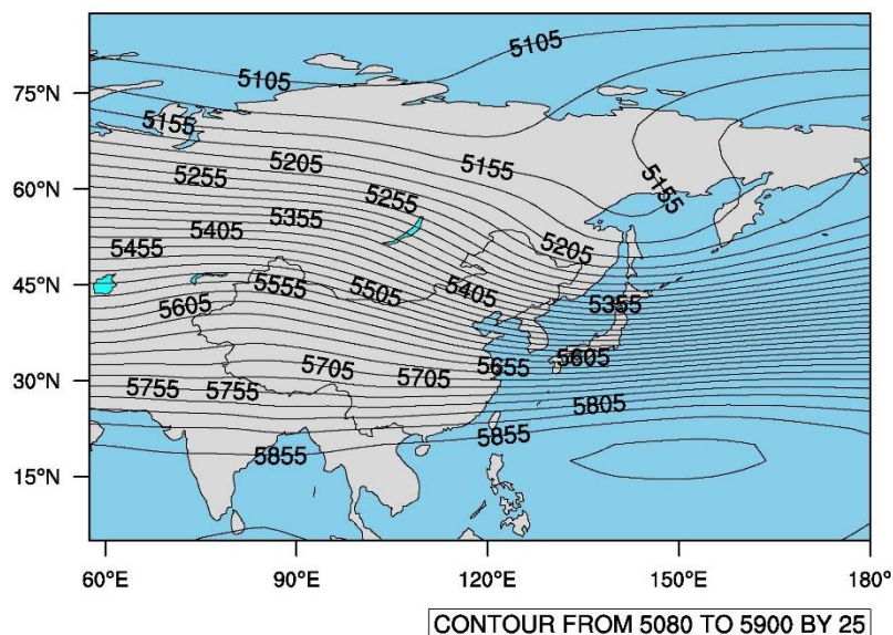
图 3.1-4 冬季 500hPa 平均环流场(1990-2019 年)
