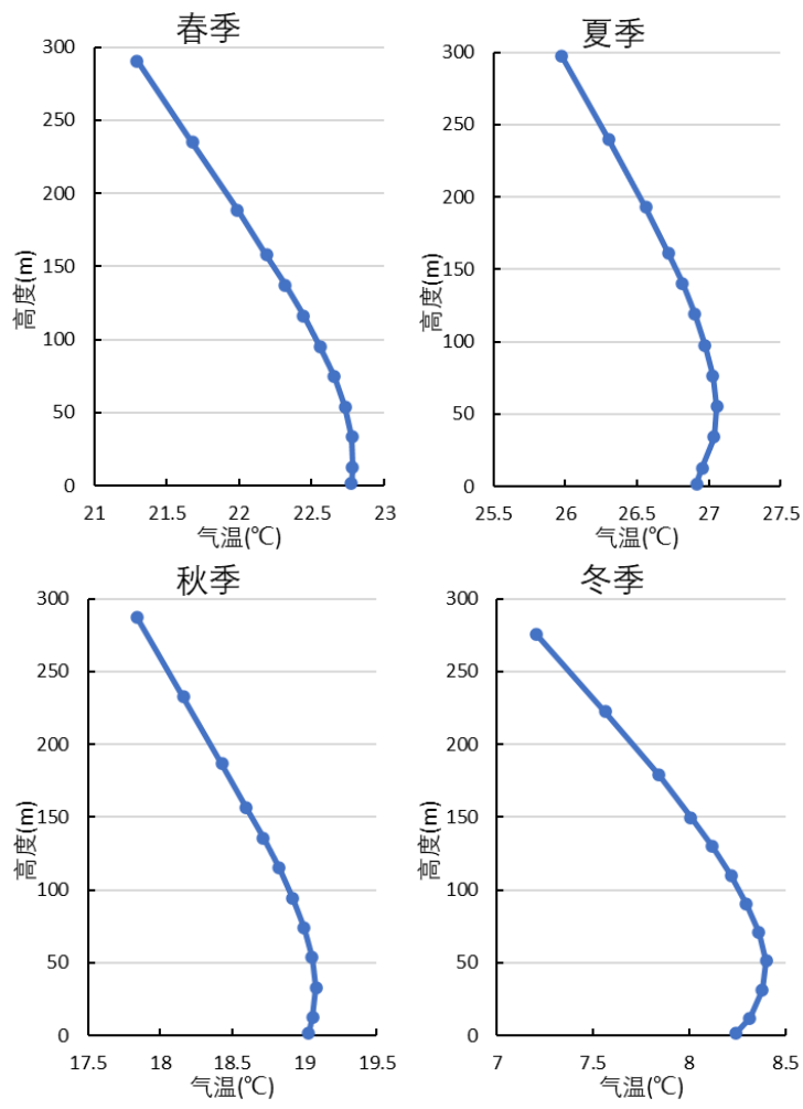
图 5.3-8 西彭工业园区春、夏、秋、冬平均气温随高度变化曲线
