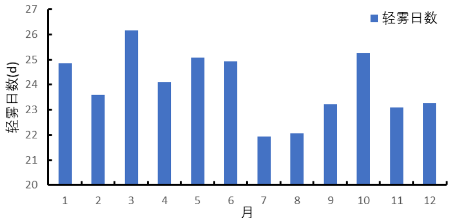
图 4.8-2 参证站轻雾平均日数年变化(1973~2019 年)
