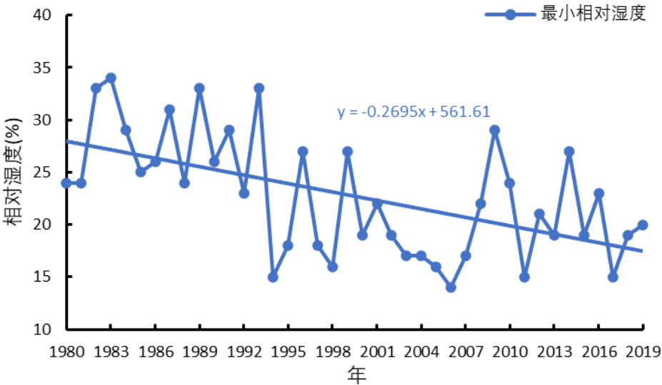
图 3.4-2 参证站最小相对湿度年际变化(1980~2019 年)
