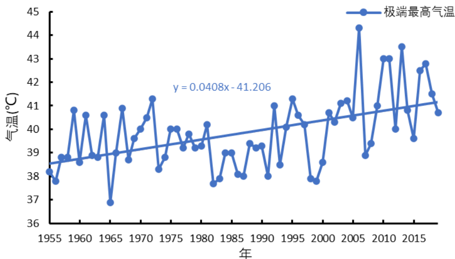
图 3.3-3 参证站极端最高气温年际变化(1955~2019 年)
