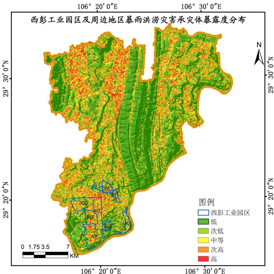
图 6.3-2 西彭工业园区及周边地区暴雨灾害承灾体暴露度分布
