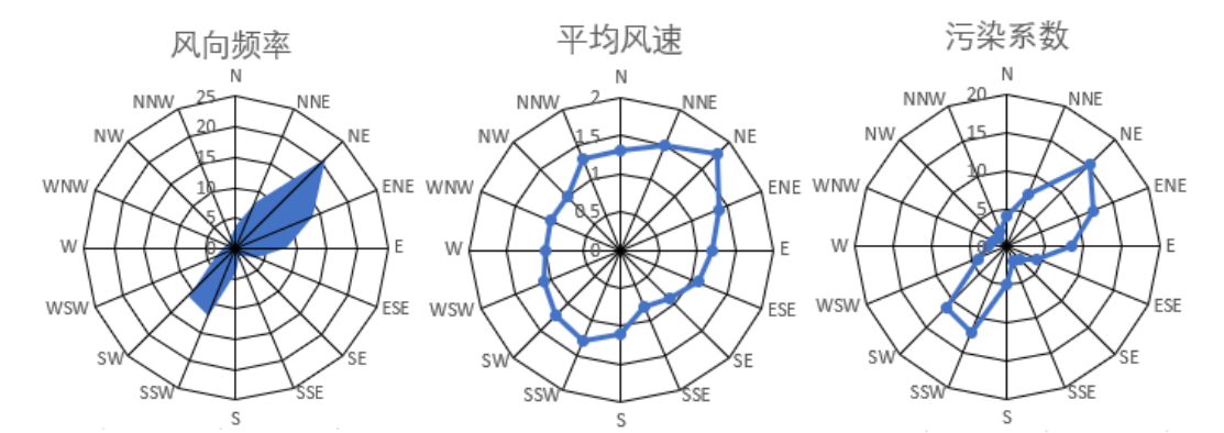
图 5.7-4 冬季风向频率、平均风速及污染系数分布(2010~2019 年)
