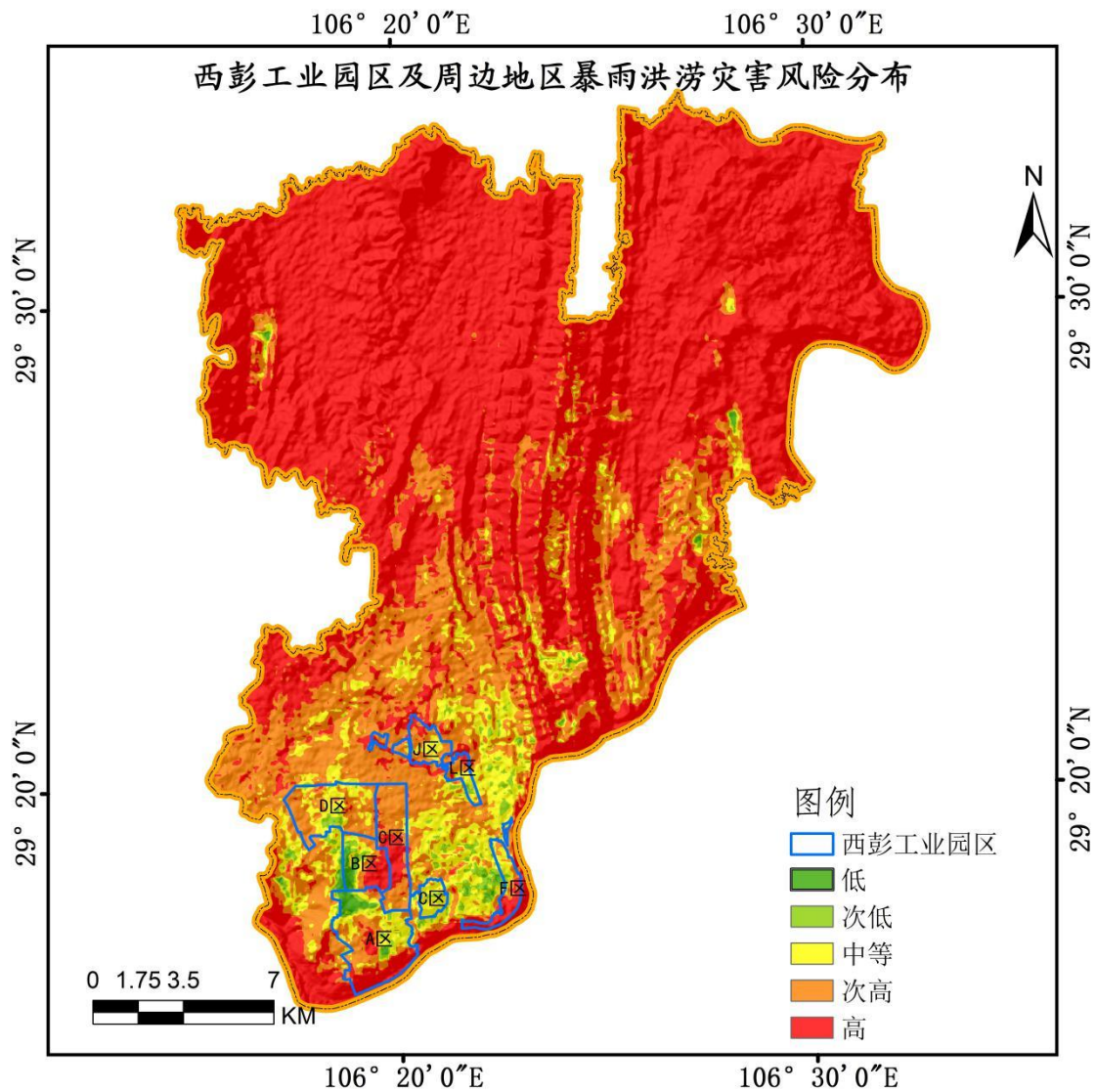
图 6.3-5 西彭工业园区及周边地区暴雨灾害风险分布
