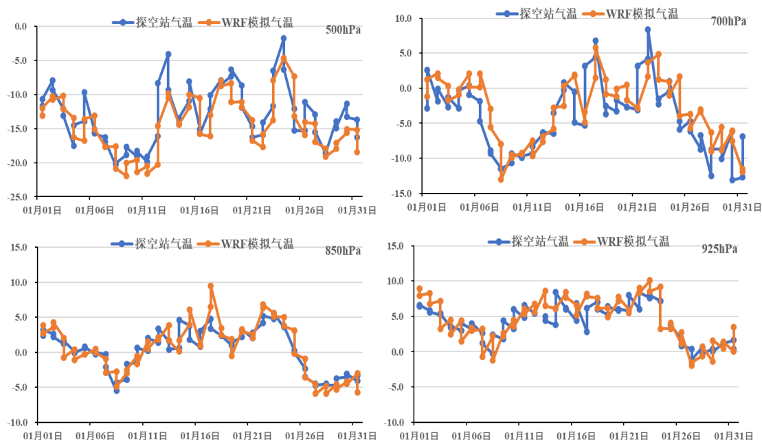
图 5.3-4 1 月模拟气温与探空站气温对比
