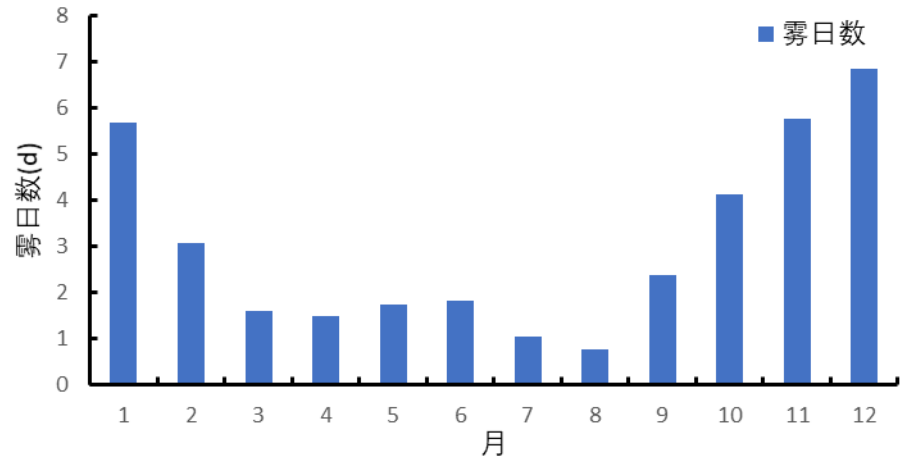
图 4.8-4 参证站雾平均日数年变化(1973~2019 年)
