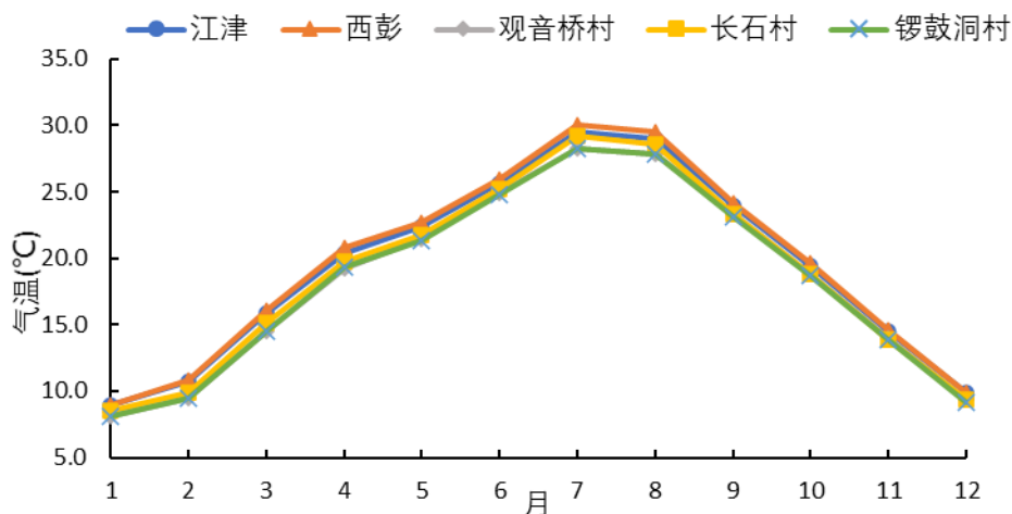
图 2.4-1 江津气象站与周边区域自动站平均气温年变化(2013~2019 年)
