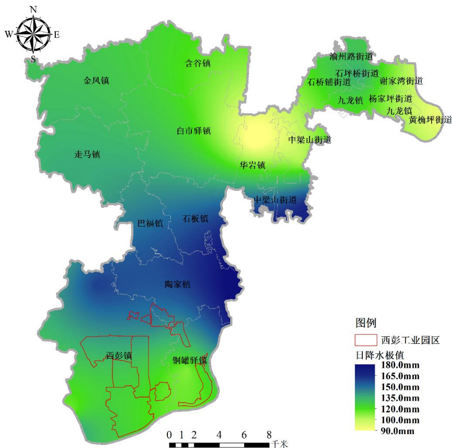
图 4.3-2 九龙坡日降水极值空间分布图(2013~2019 年)
