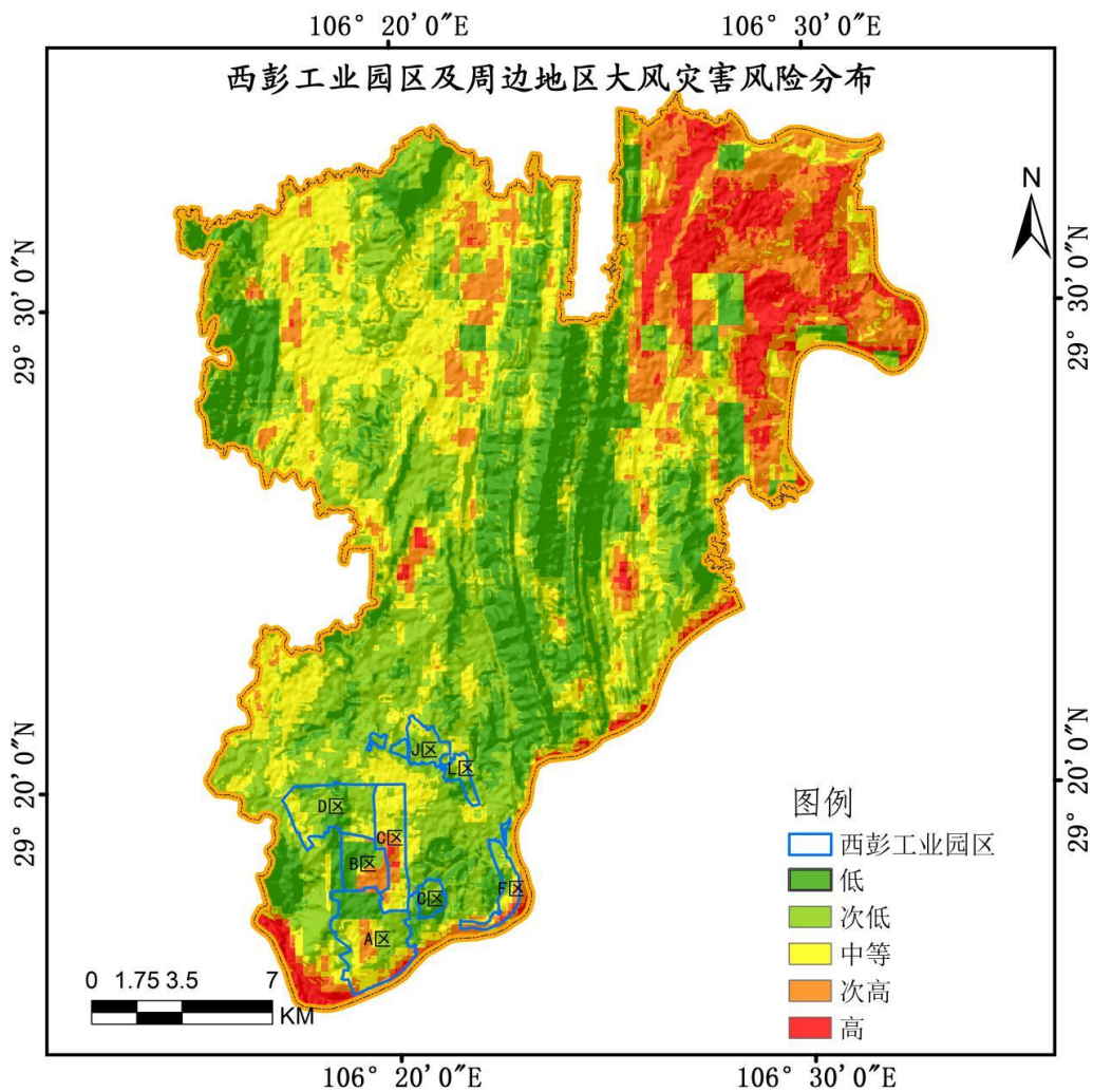
图 6.2-5 西彭工业园区及周边地区大风灾害风险分布
