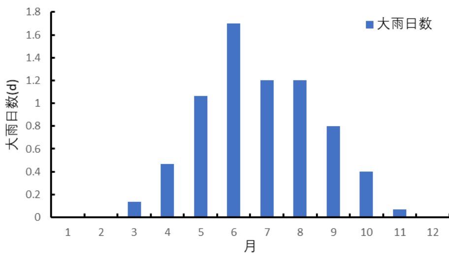
图 3.5-7 参证站大雨日数年变化(1990~2019 年)
