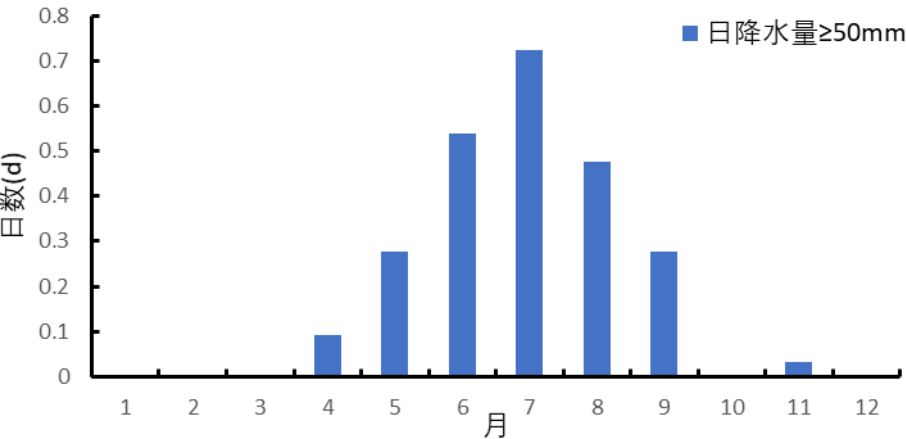
图 5.4-2b 日降水量 \geq 50.0\text{mm} 平均日数的年变化(1955~2019 年)
