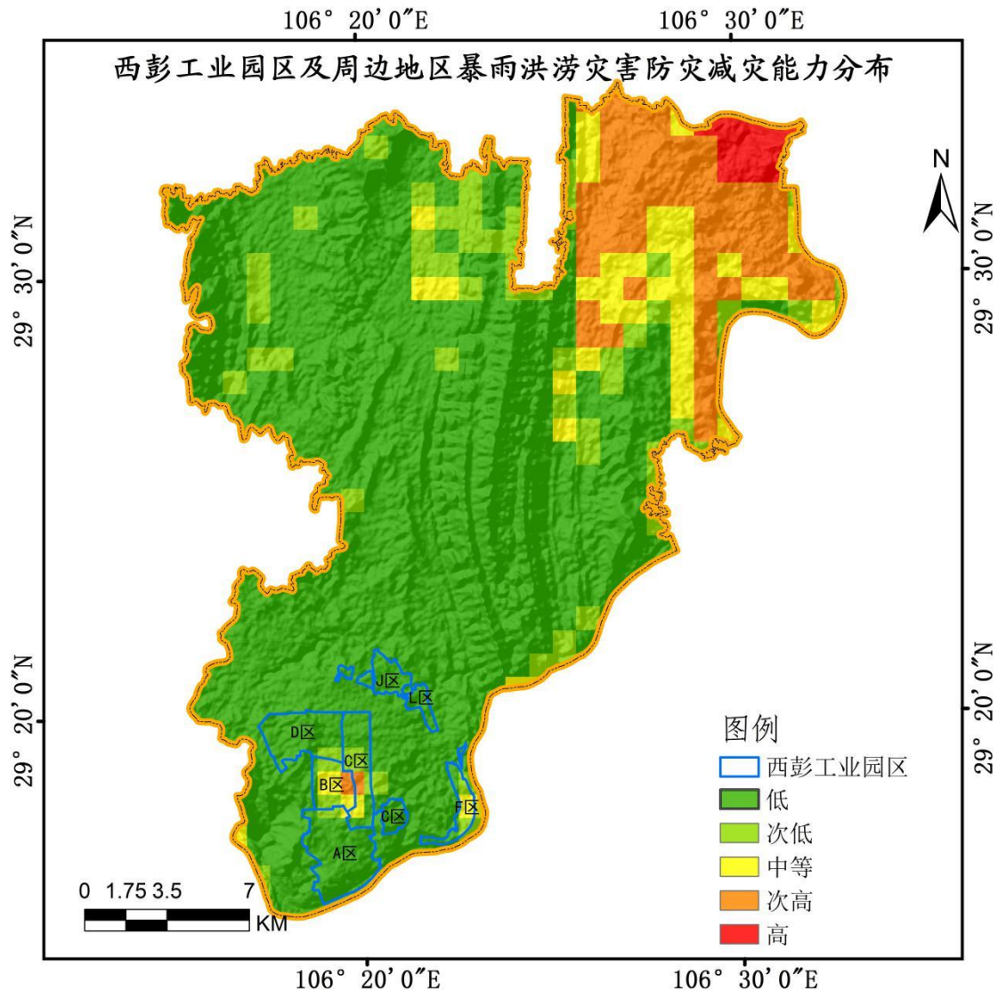
图 6.3-4 西彭工业园区及周边地区暴雨灾害防灾减灾能力分布
