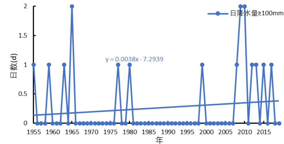
图 5.4-3a 日降水量≥100.0mm 日数的年际变化(1955~2019 年)
