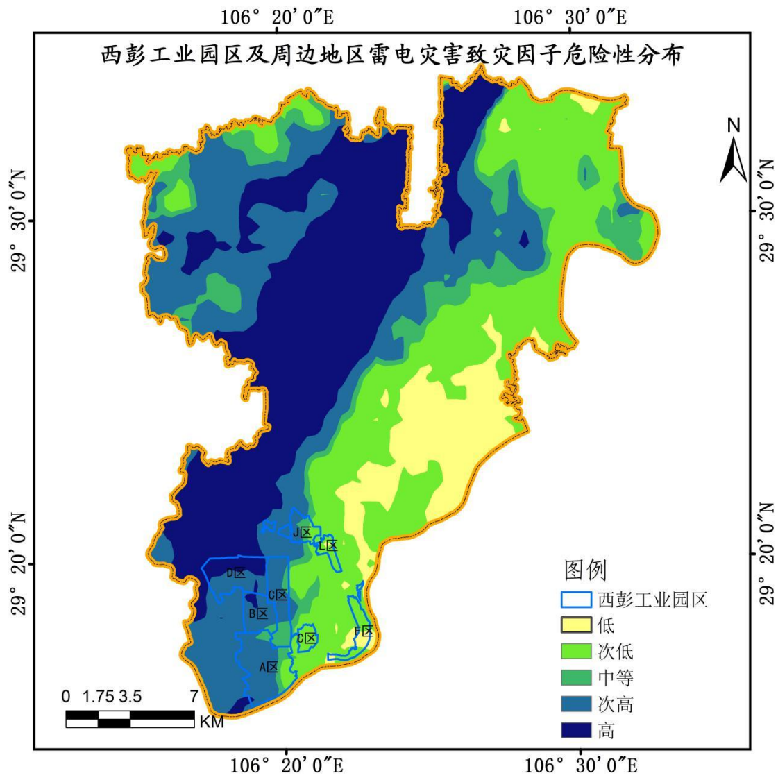
图 6.4-13 西彭工业园区及周边地区雷电致灾因子危险性分布
