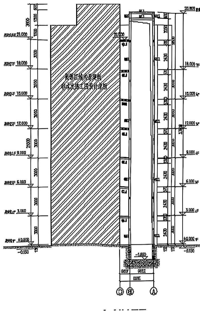
图 2-2 新增电梯标准层结构立面布置
