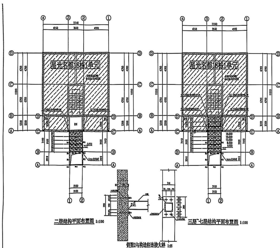
图 2-1 新增电梯标准层结构平面布置
