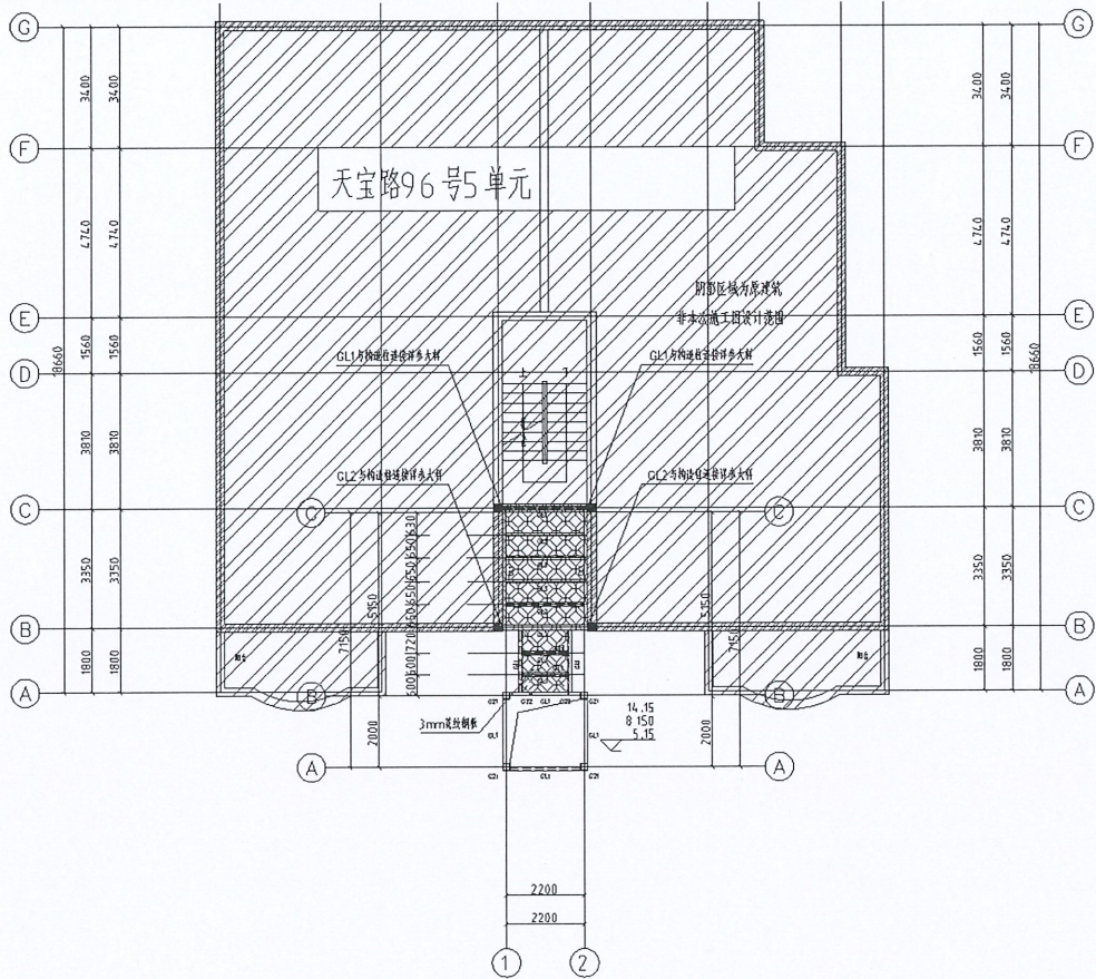
图 3.2.1 新增电梯平面示意图
