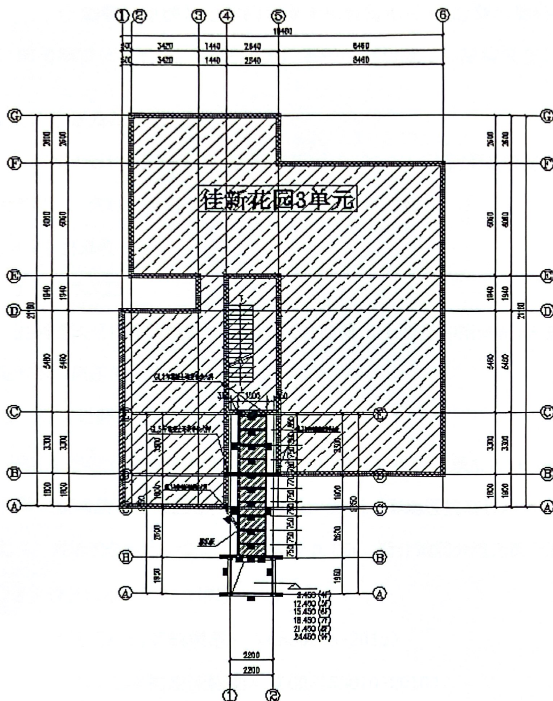
图 2-1 新增电梯标准层结构平面布置
