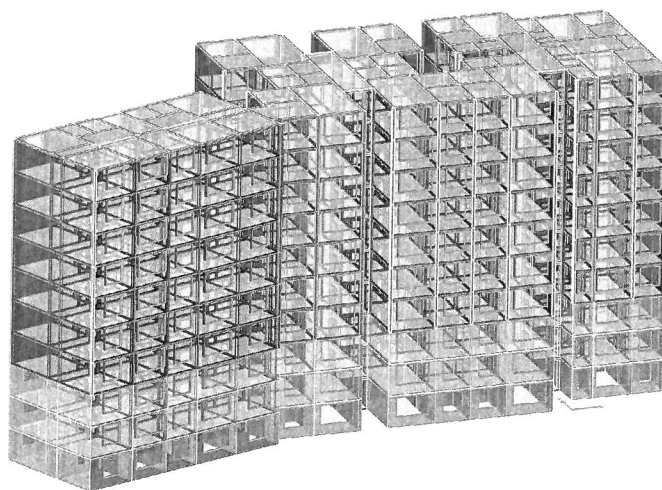
图 4-1 结构三维模型图
