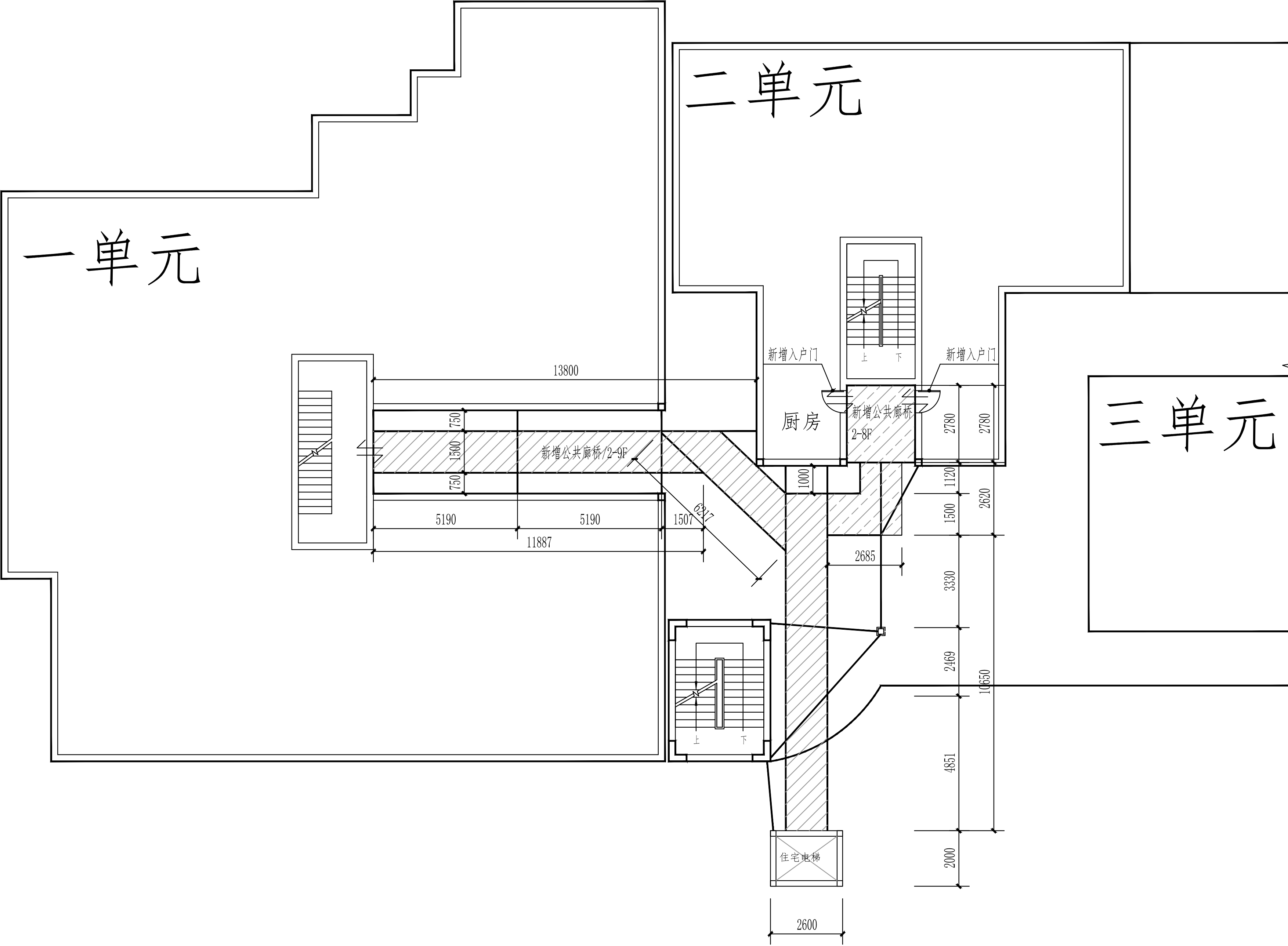
住宅标准层--九龙坡区兴胜路61号增设电梯示意图
