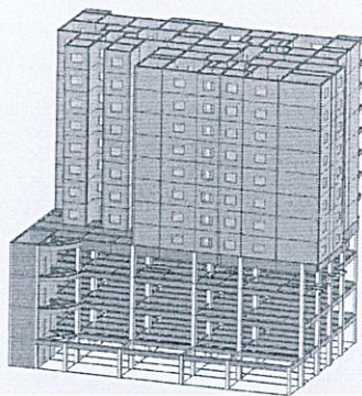
图 1 结构三维模型
